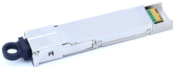
图10-2 10G EPON OLT 光模块（SC 接口）外观示意图
