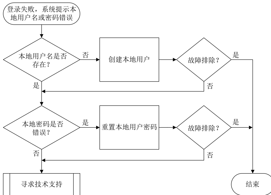
图15-5 本地用户名或密码错误的故障诊断流程图
