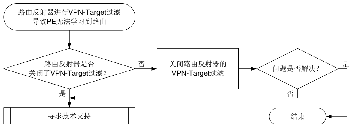
图10-11 路由反射器进行 VPN-Target 过滤导致 PE 无法学习到路由故障处理流程
