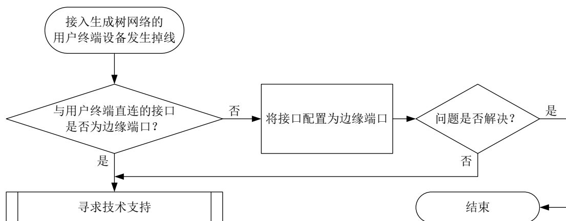
图6-2 接入生成树网络的用户终端设备发生掉线的故障诊断流程图
