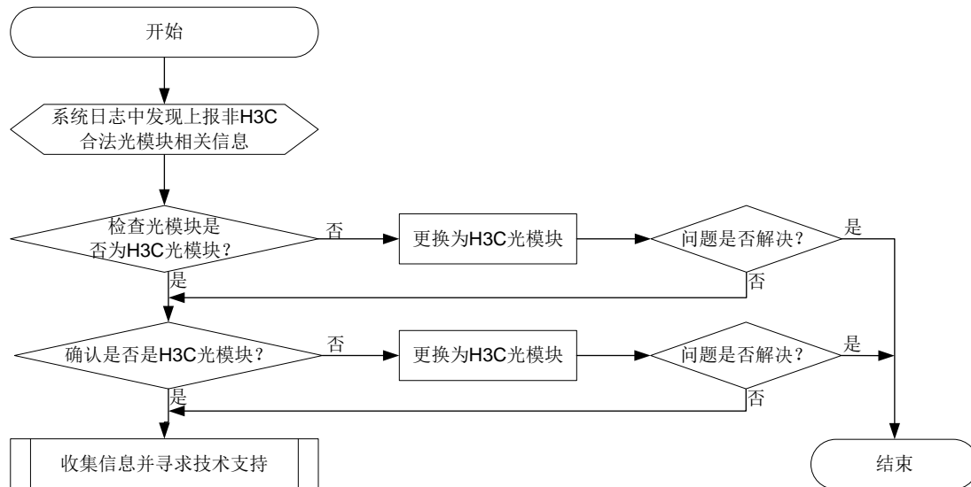
图2-22 故障诊断流程图
