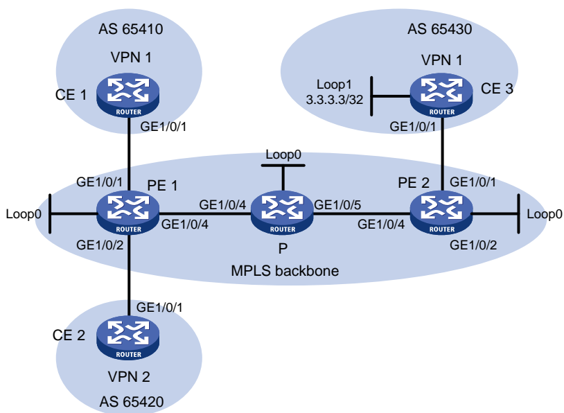
图10-9 MPLS L3VPN 组网图
