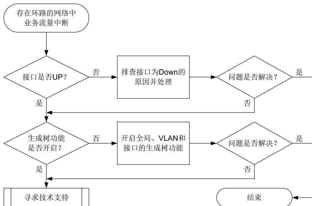
图6-1 设备连接成环时业务中断的故障诊断流程图
