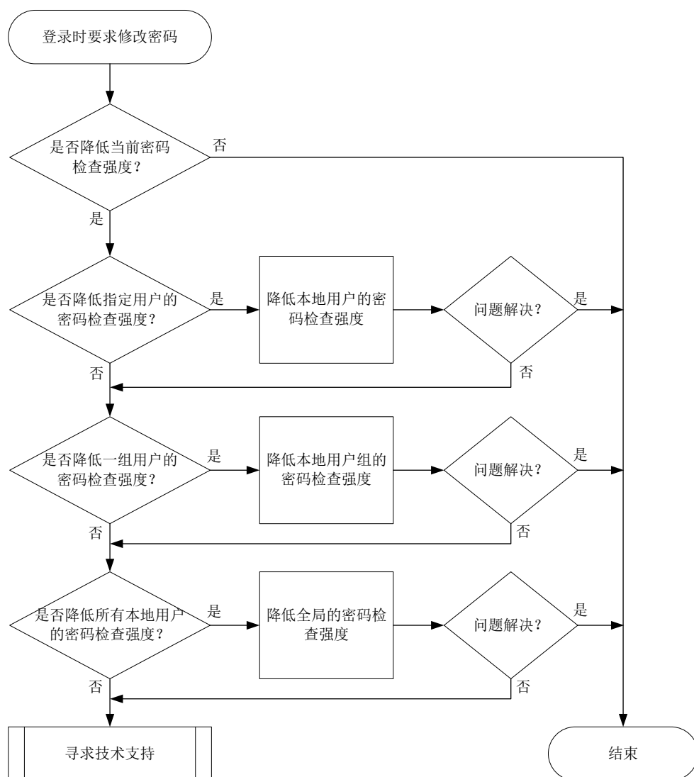
图15-18 管理员登录时要求修改密码故障诊断流程图
