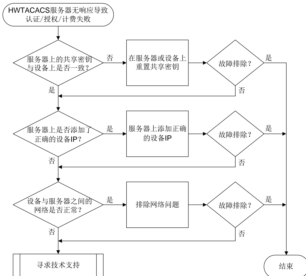
图15-12 HWTACACS 服务器无响应的故障诊断流程图
