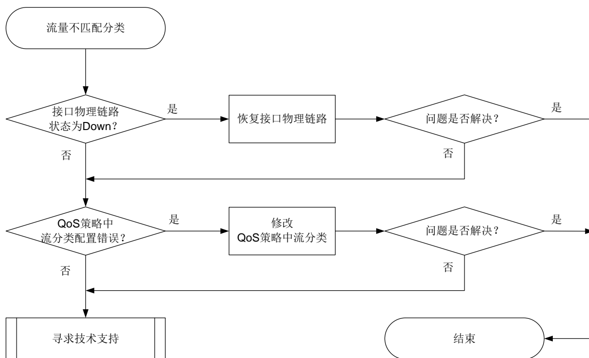
图14-1 流量不匹配分类的故障诊断流程图
