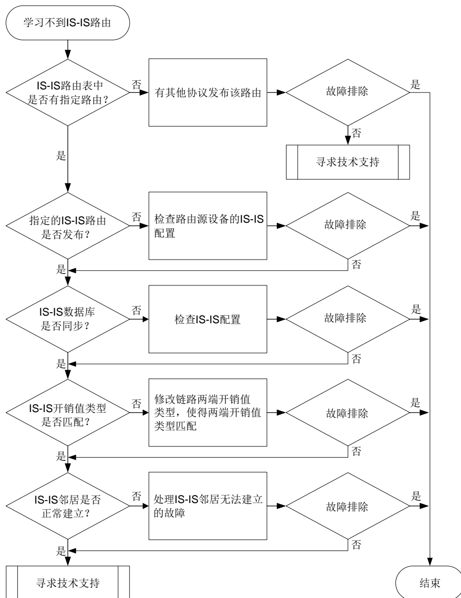
图8-4 设备学习不到IS-IS路由的故障诊断流程图
