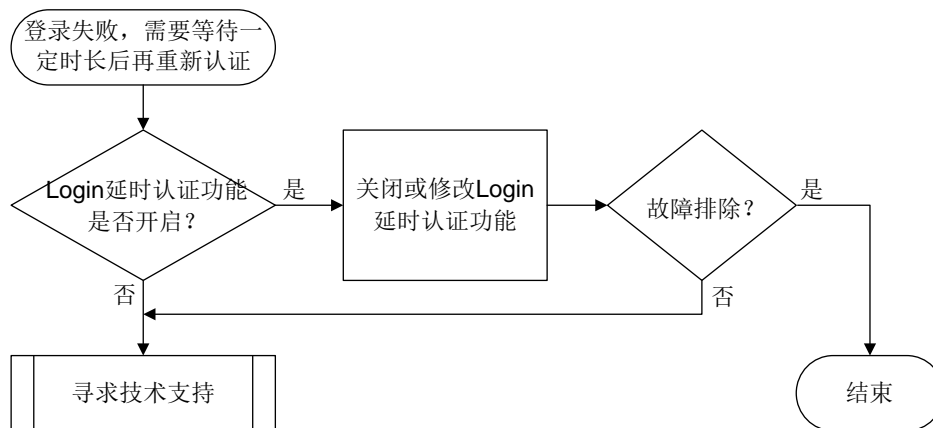
图15-8 登录失败后等待重认证的故障诊断流程图
