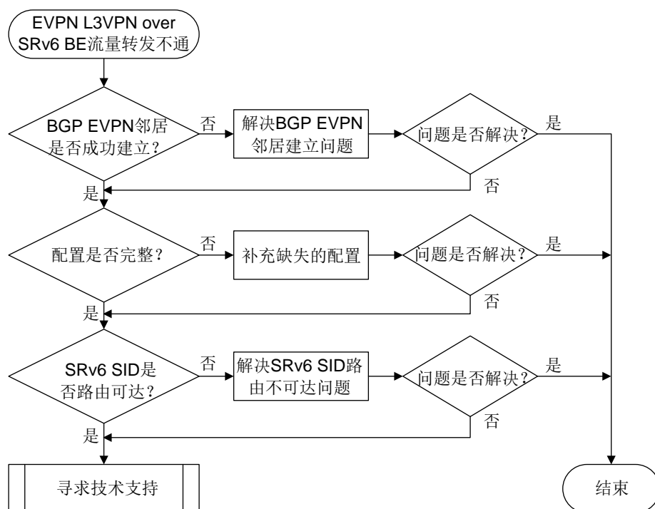
图11-1 EVPN L3VPN over SRv6 BE 流量转发不通的故障诊断流程图
