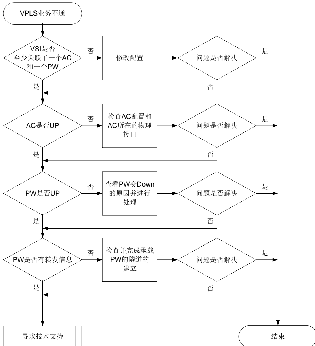
图10-21 VPLS业务不通的故障诊断流程图
