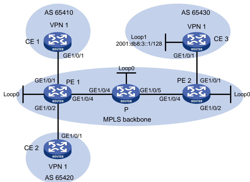
图10-14 IPv6 MPLS L3VPN 组网图
