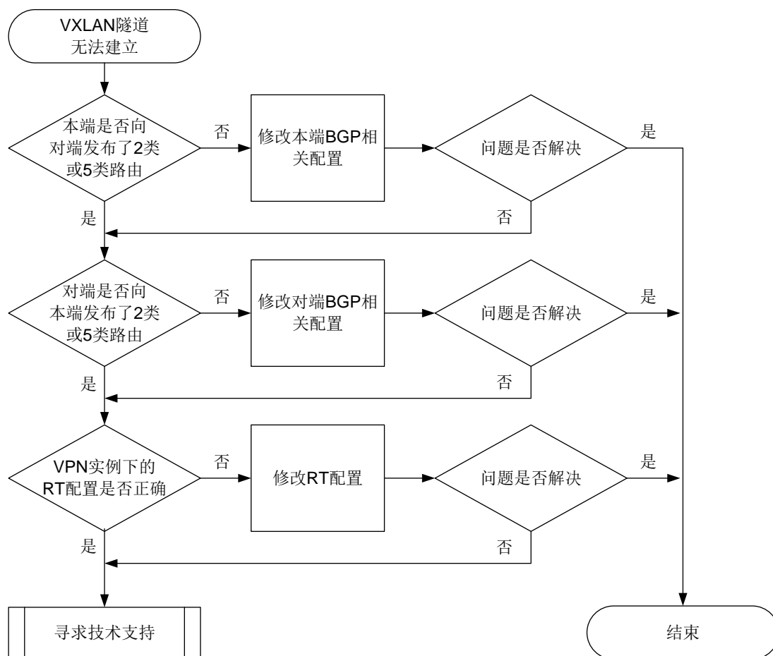
图13-2 不同 VXLAN 内 VTEP 之间的 VXLAN 隧道无法建立的故障诊断流程图
