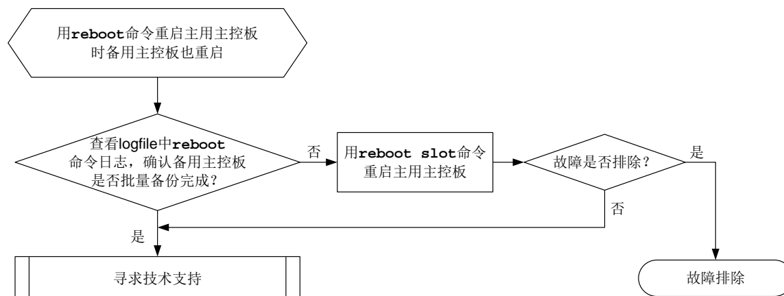
图2-13 故障诊断流程图
