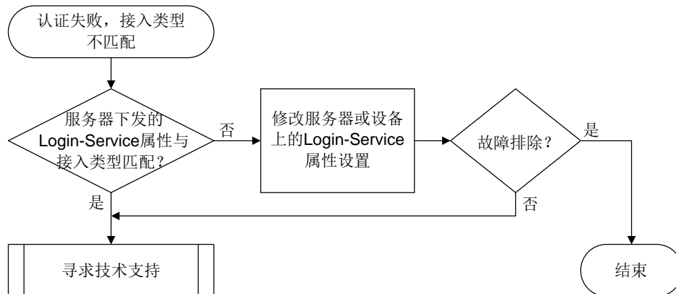
图15-13 用户接入类型与 RADIUS 服务器下发的 Login-Service 属性值不匹配的故障诊断流程图
