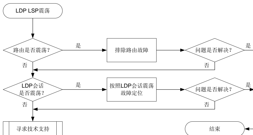
图10-4 LDP LSP 震荡的故障诊断流程图
