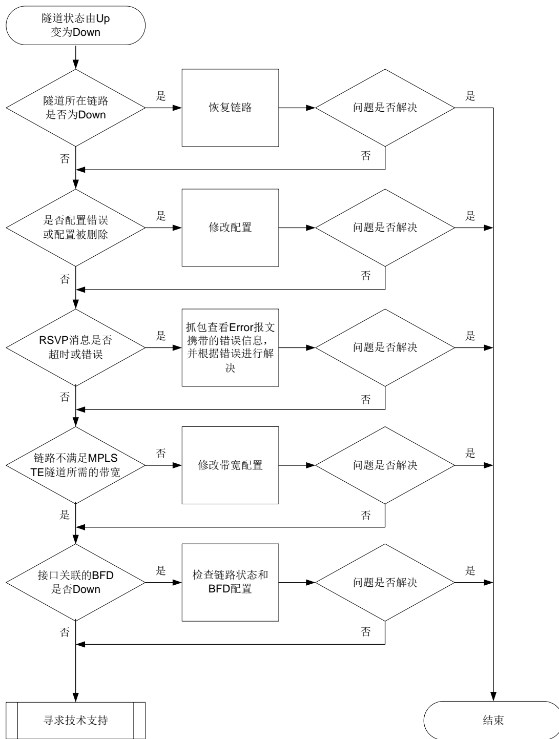
图10-17 MPLS TE 隧道由 UP 状态突然变为 Down 状态的故障诊断流程图
