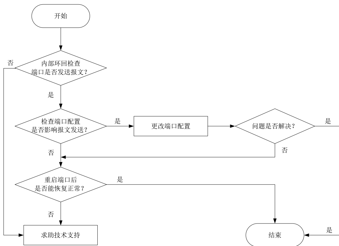
图2-18 故障诊断流程图
