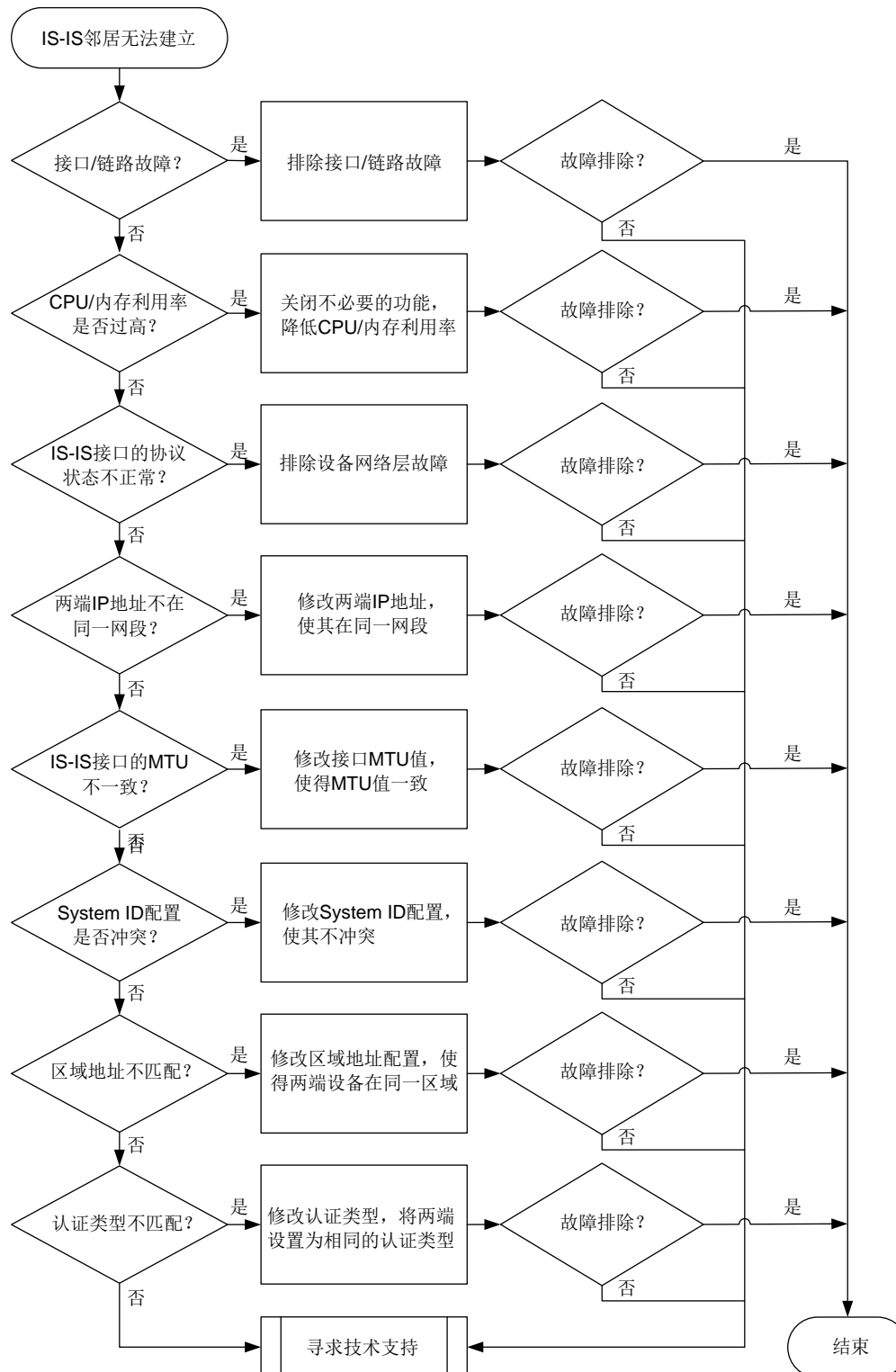
图8-3 IS-IS 邻居无法建立的故障诊断流程图
