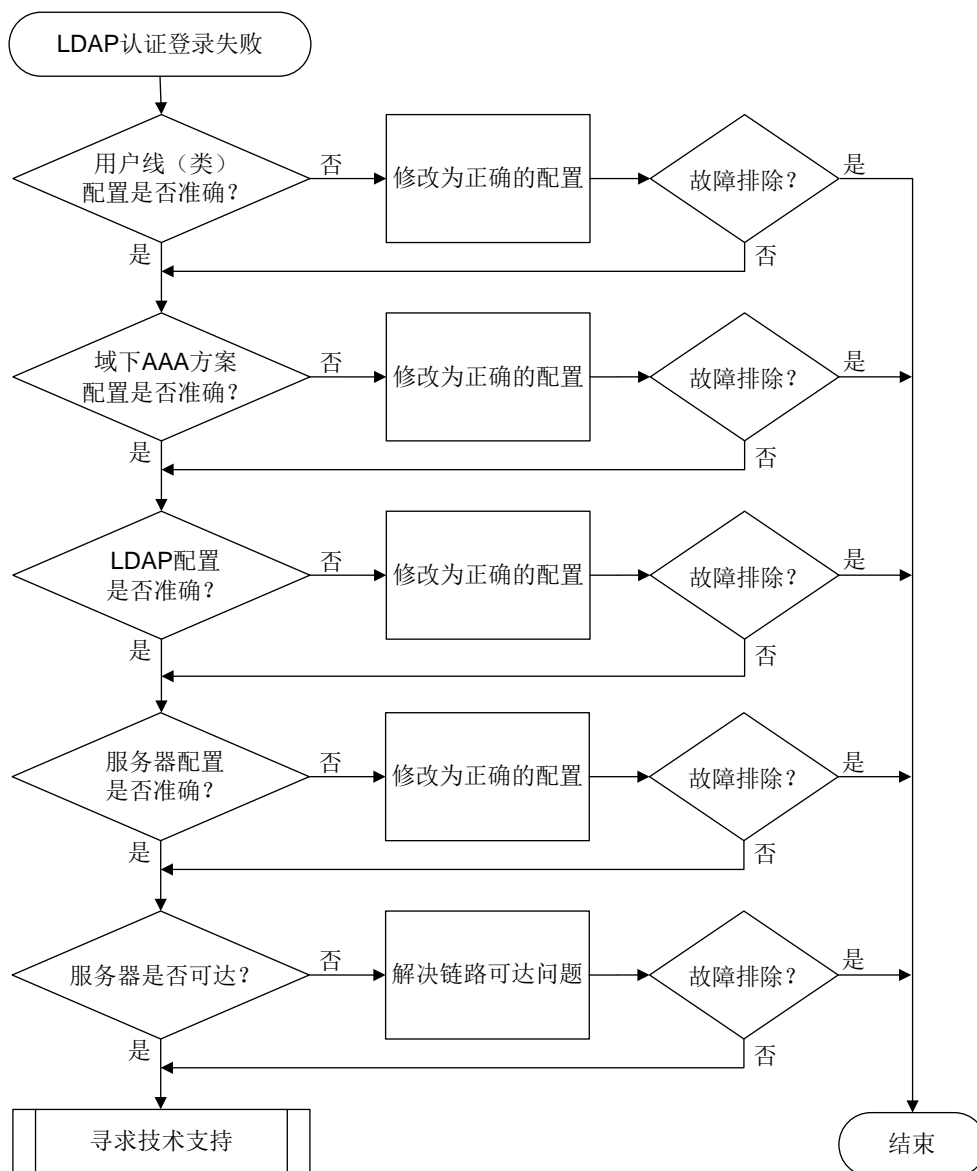
图15-17 LDAP 认证登录失败的故障诊断流程图
