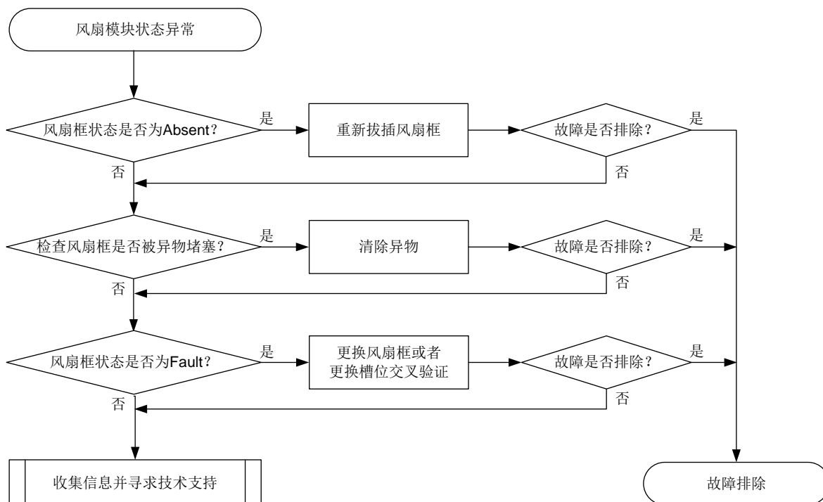
图2-8 故障诊断流程图
