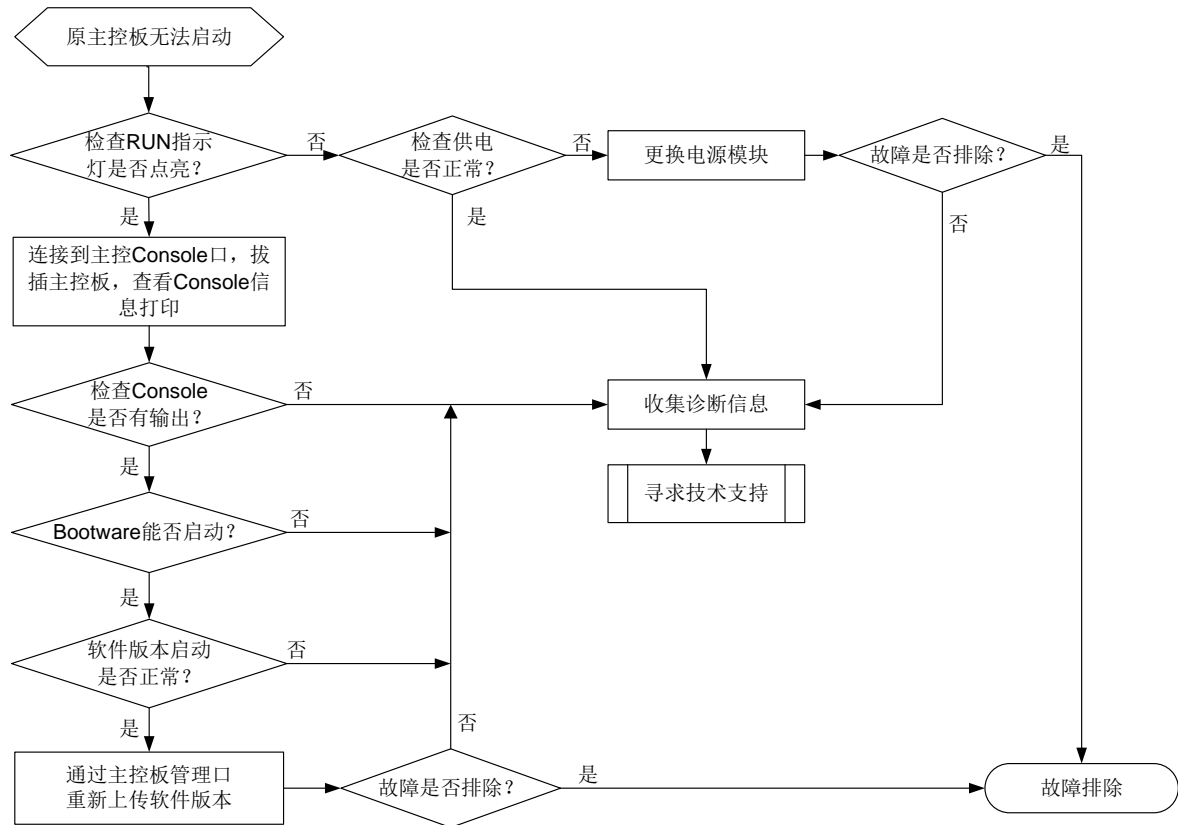
图2-10 原主控板无法启动故障诊断流程图
