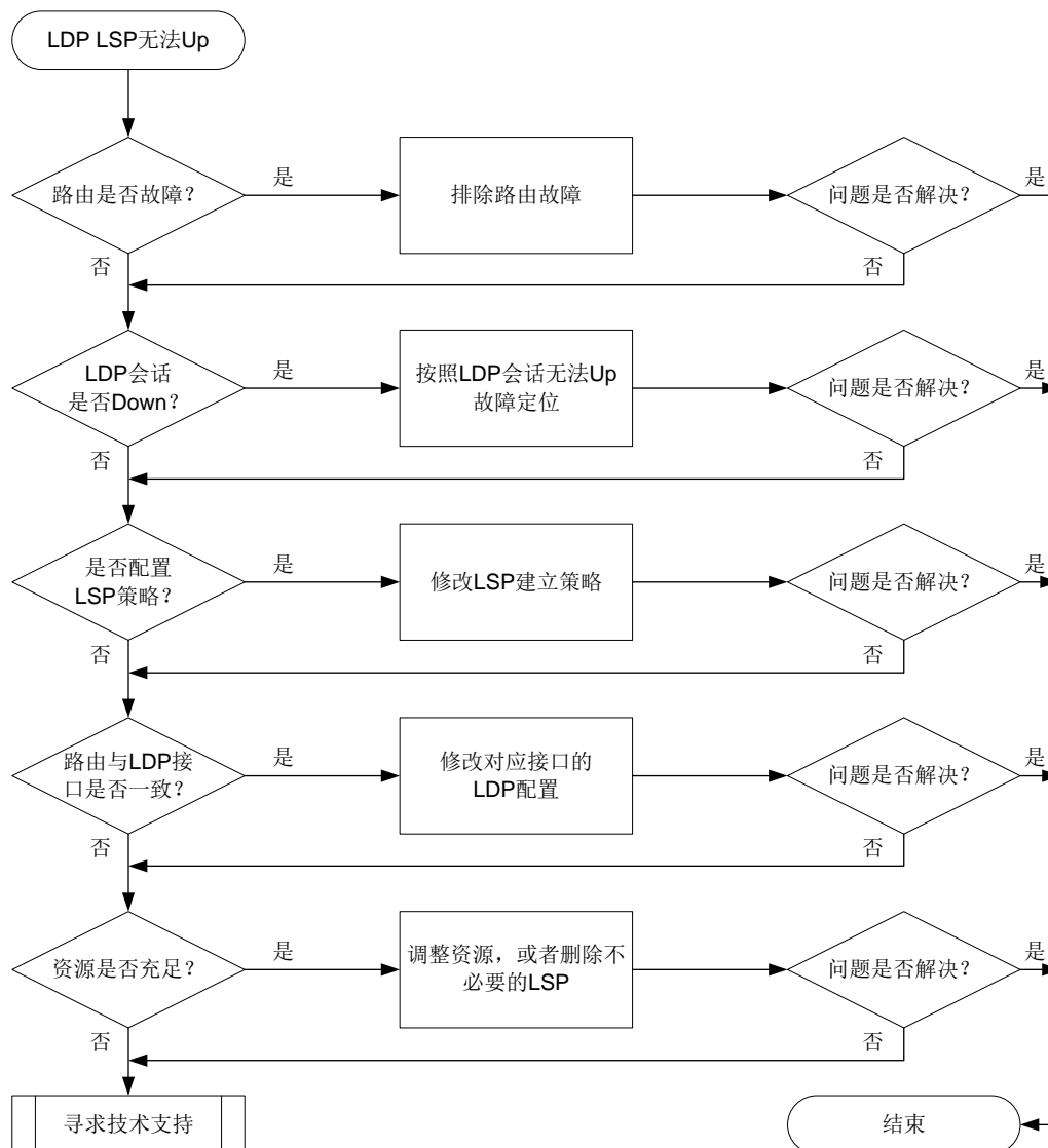
图10-3 LDP LSP Down 的故障诊断流程图
