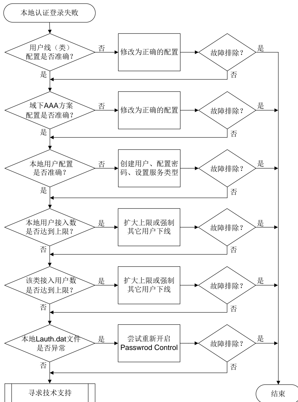
图15-14 本地认证登录失败的故障诊断流程图
