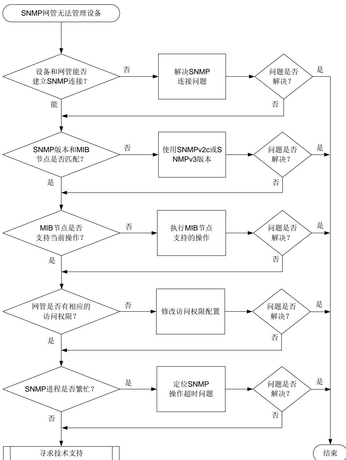
图18-5 网管无法管理设备的故障诊断流程图
