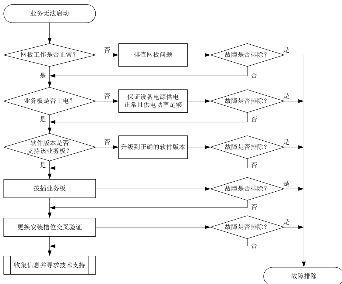
图2-14 故障诊断流程图
