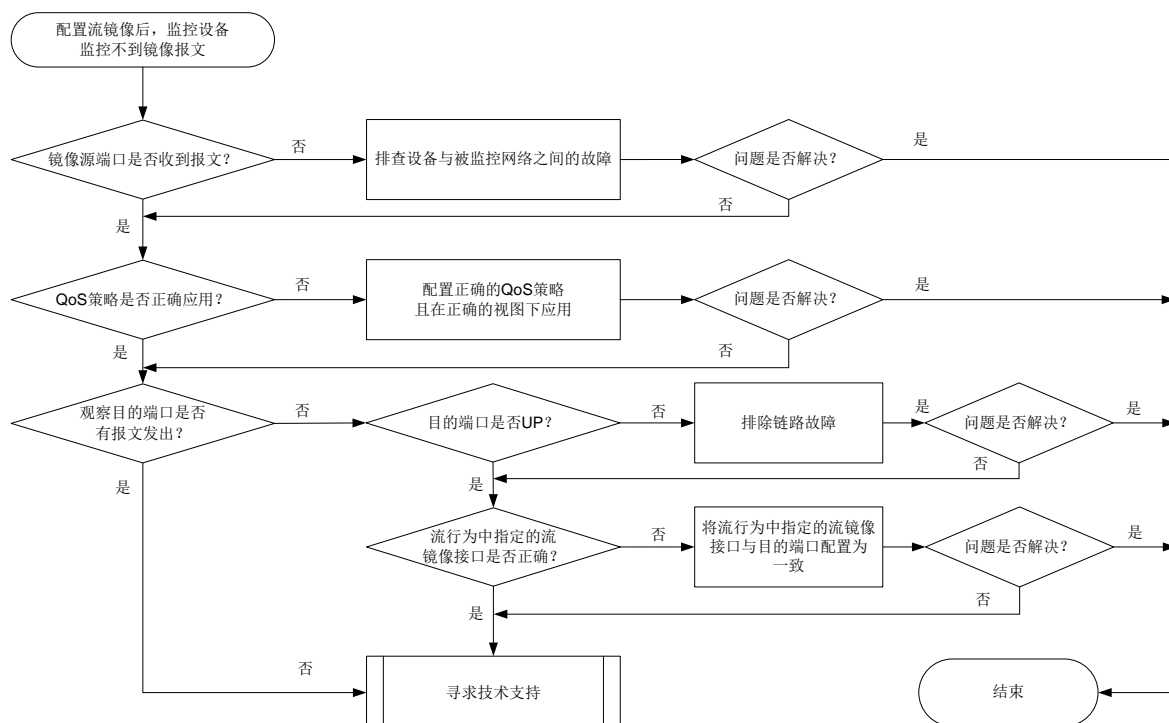
图18-7 配置流镜像后监控设备收不到镜像报文的故障诊断流程图
