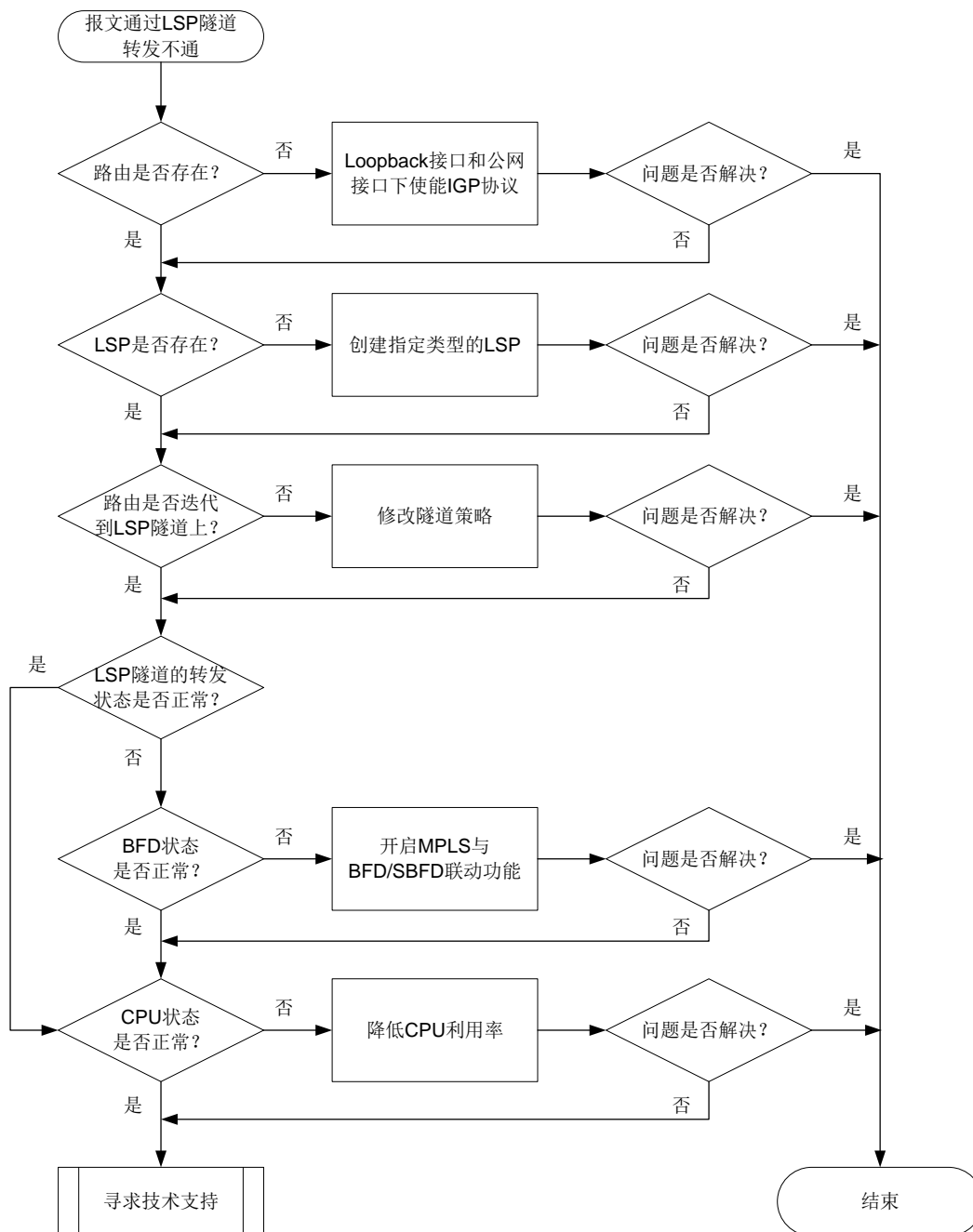
图10-20 报文通过 LSP 隧道转发不通的故障诊断流程图
