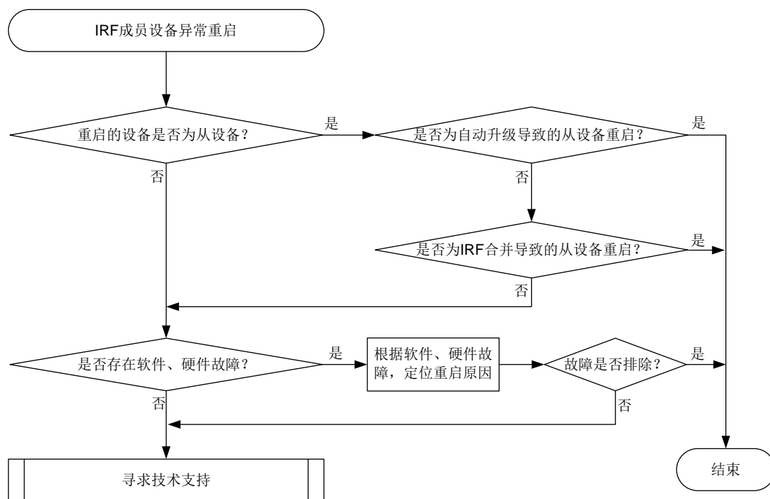
图5-2 IRF 成员设备异常重启故障诊断流程图
