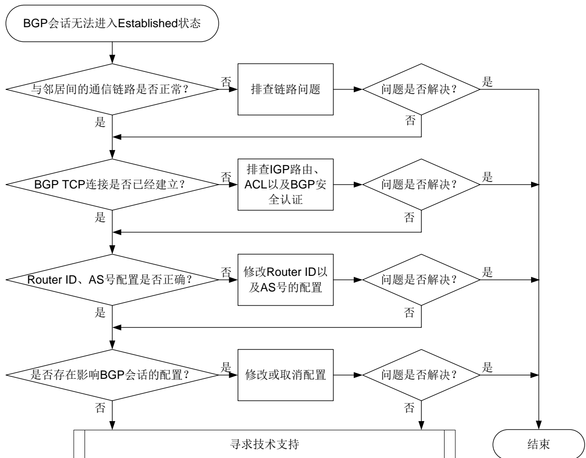
图8-1 BGP 会话无法进入 Established 状态的故障诊断流程图
