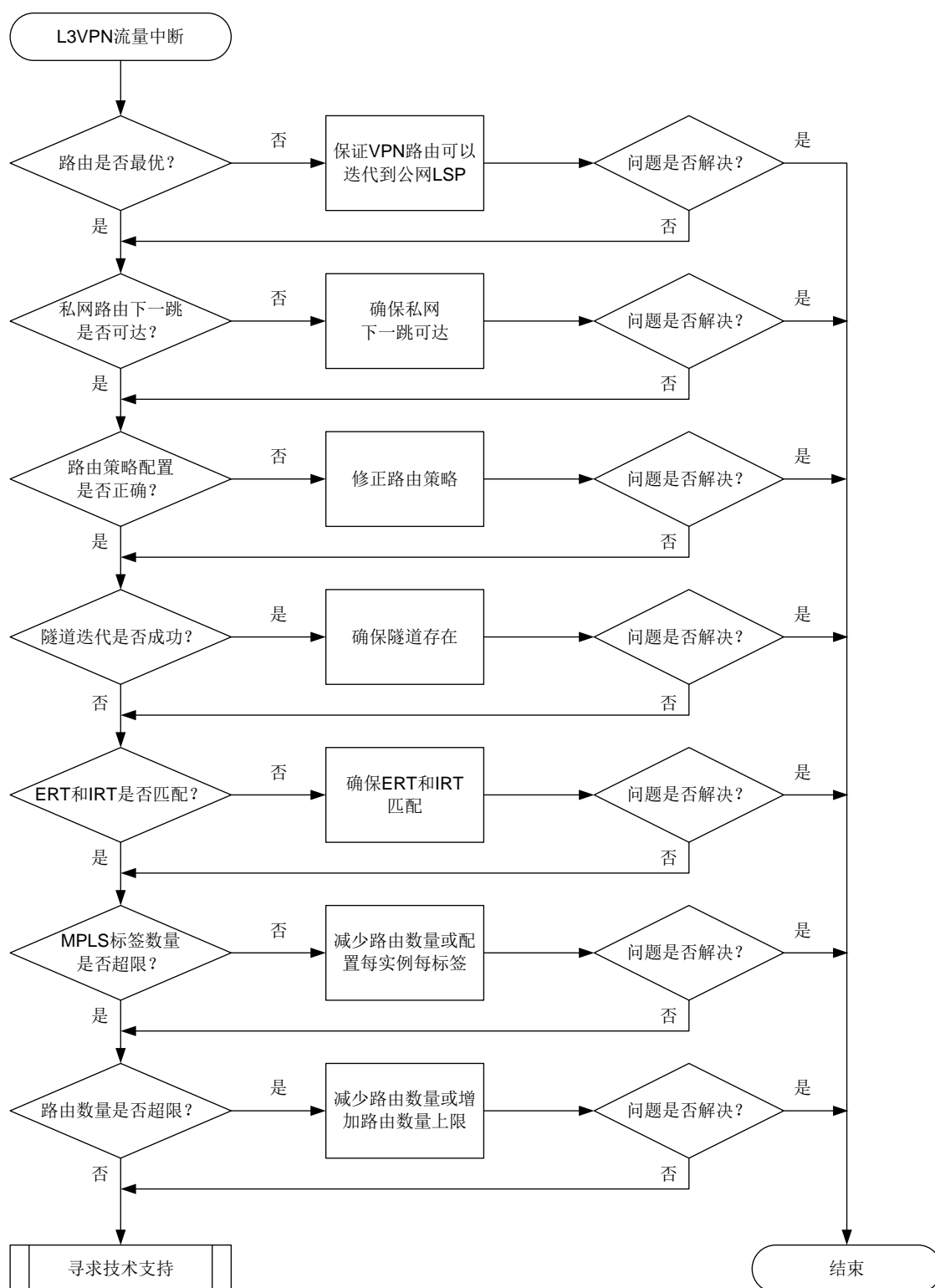
图10-6 L3VPN 流量中断故障诊断流程图
