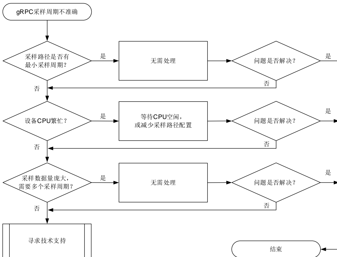
图19-1 gRPC 采样周期不准确的故障诊断流程图
