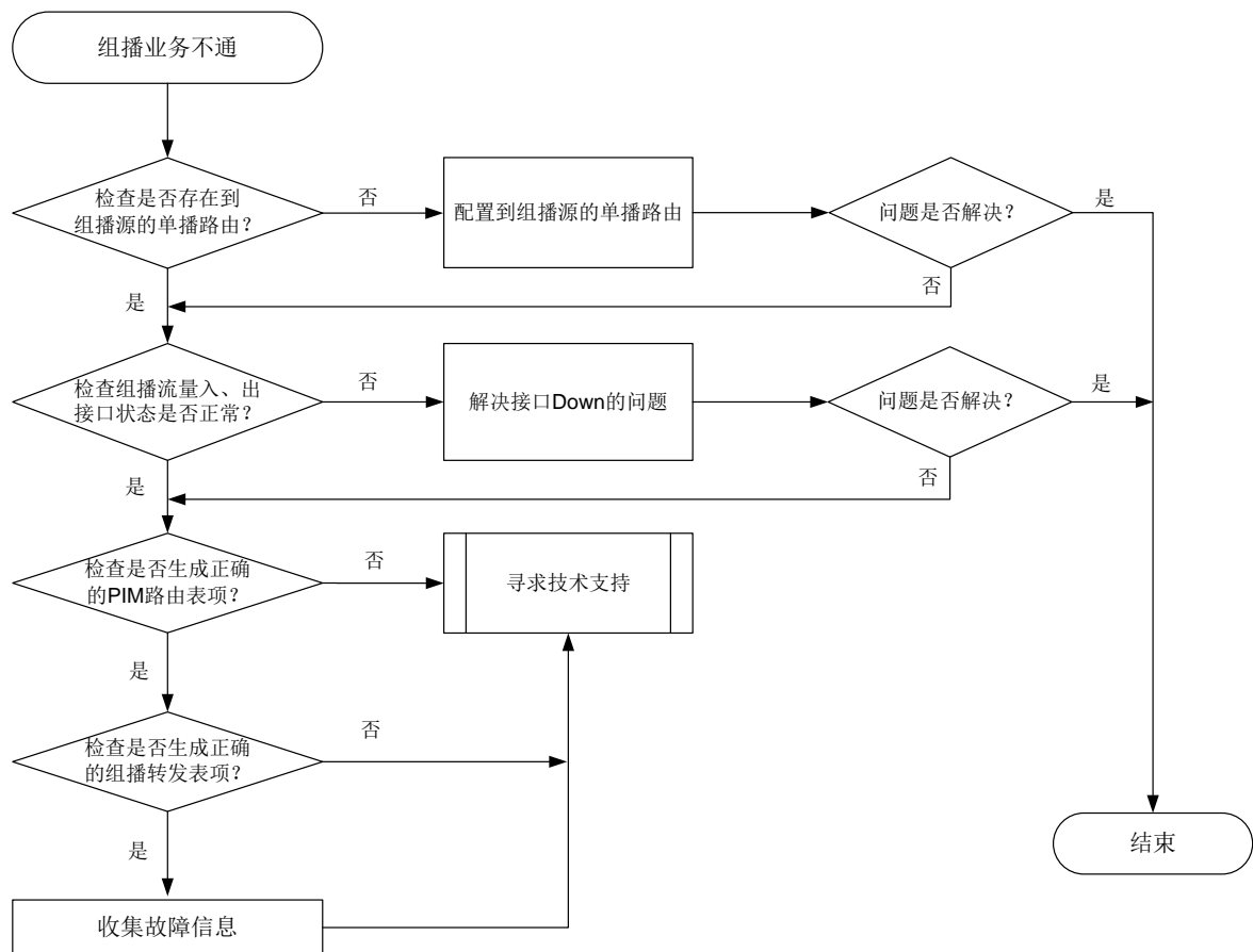
图9-7 三层组播业务不通的故障诊断流程图
