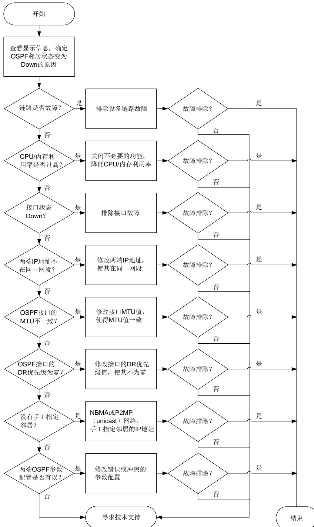
图8-8 OSPF 邻居 Down 的故障诊断流程图
