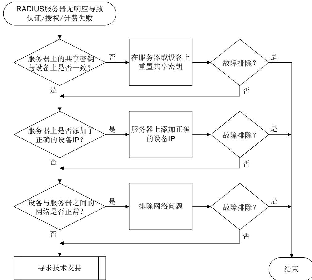
图15-11 RADIUS 服务器无响应的故障诊断流程图
