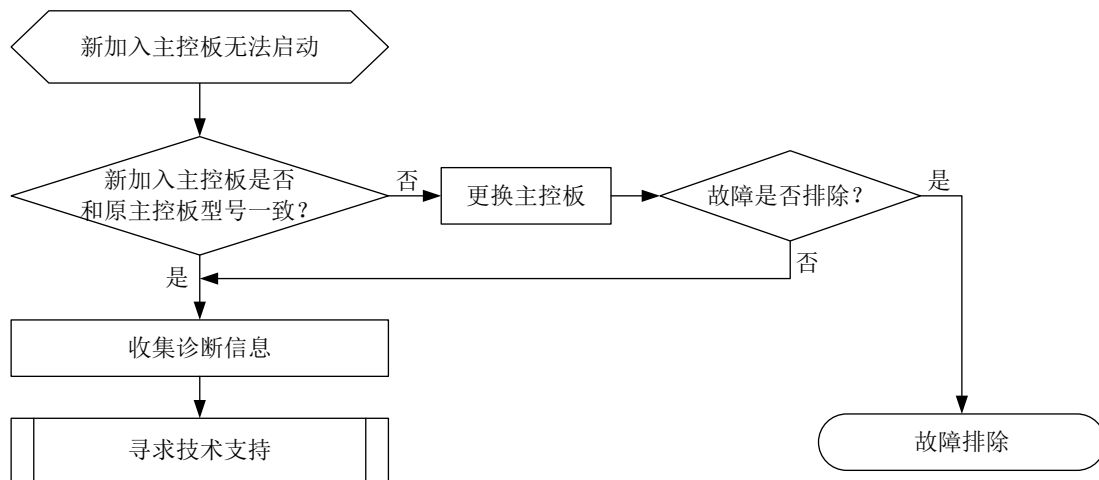
图2-11 新加入设备的备用主控板无法启动故障诊断流程图
