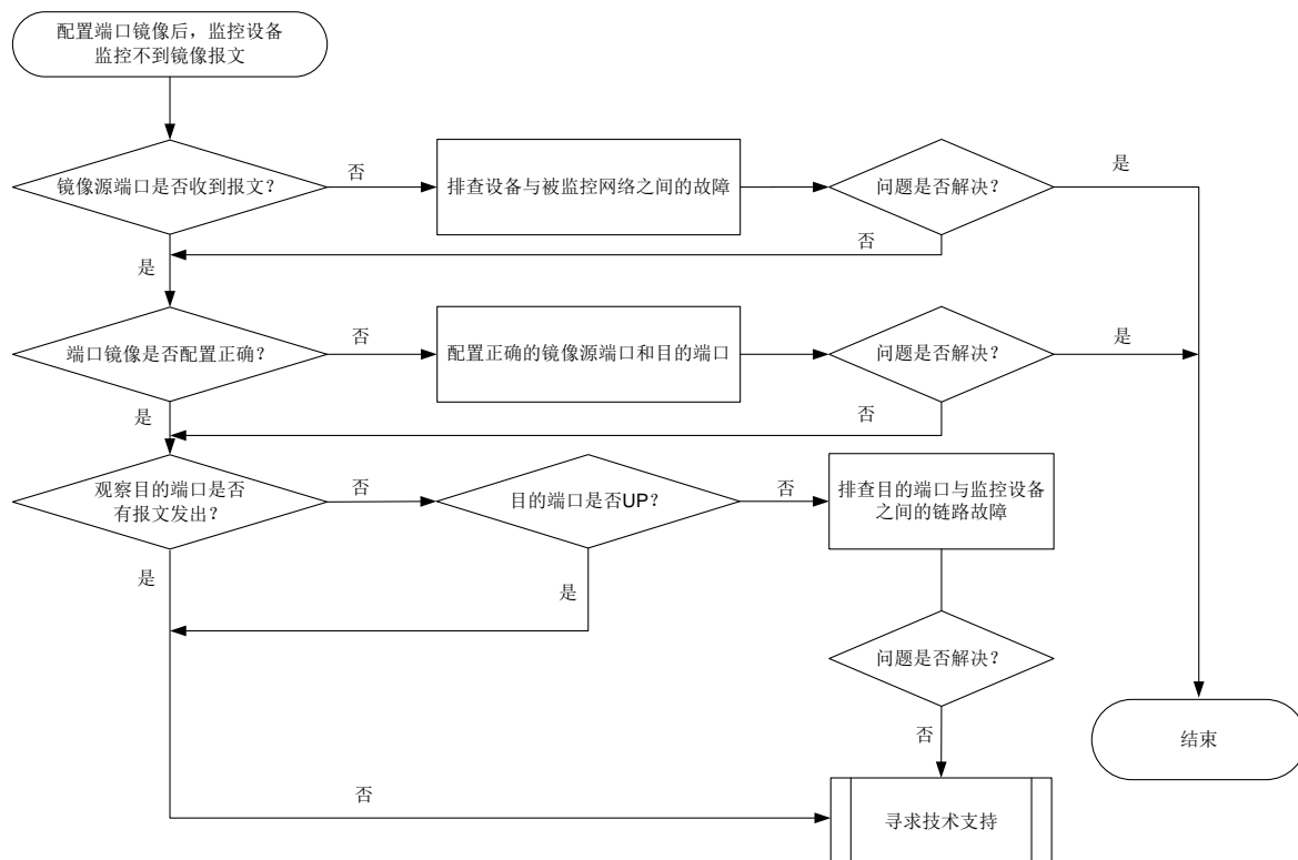
图18-8 端口镜像后监控设备收不到镜像报文的故障诊断流程图
