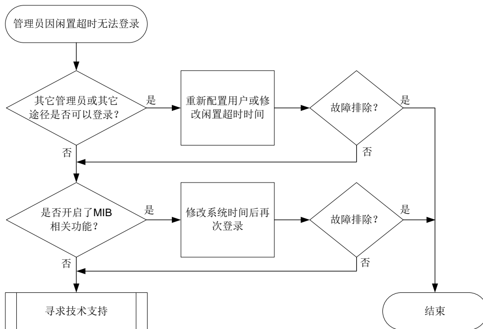
图15-20 管理员因闲置超时无法登录故障诊断流程图
