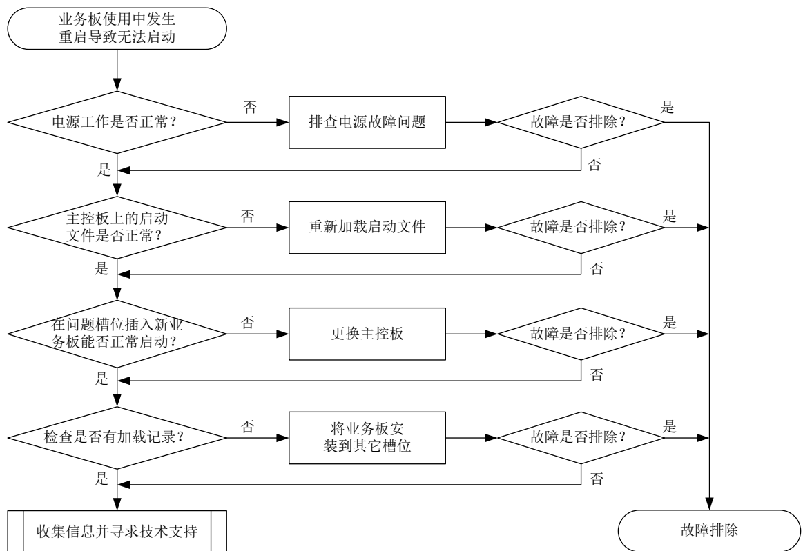
图2-15 故障诊断流程图
