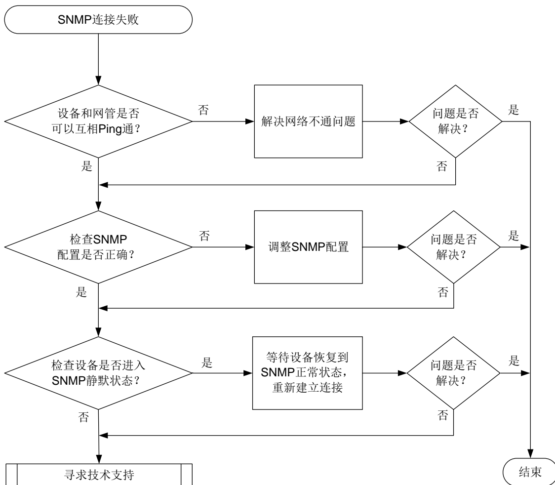
图18-3 SNMP 无法连接的故障诊断流程图
