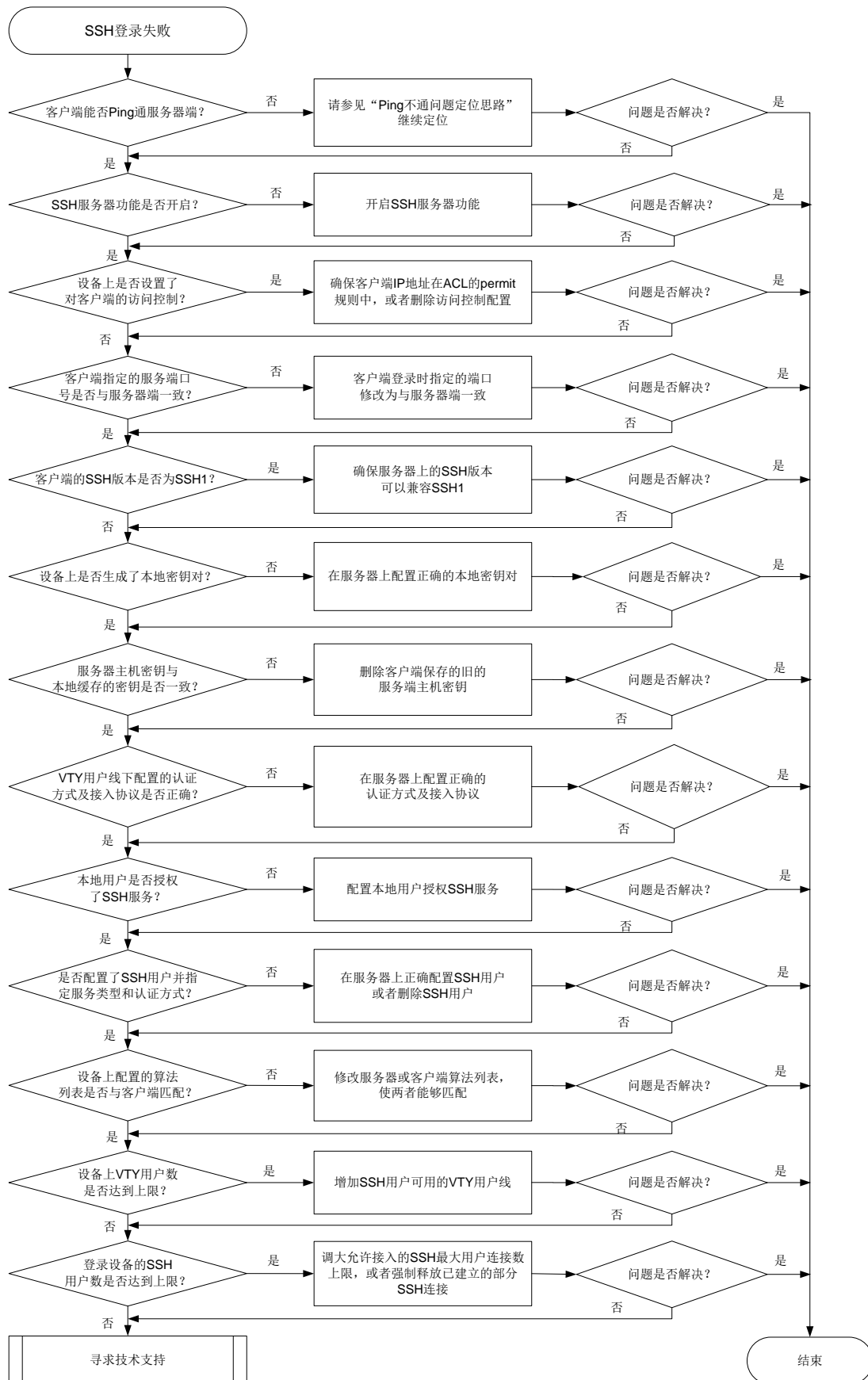
图16-1 SSH 登录失败故障诊断流程图
