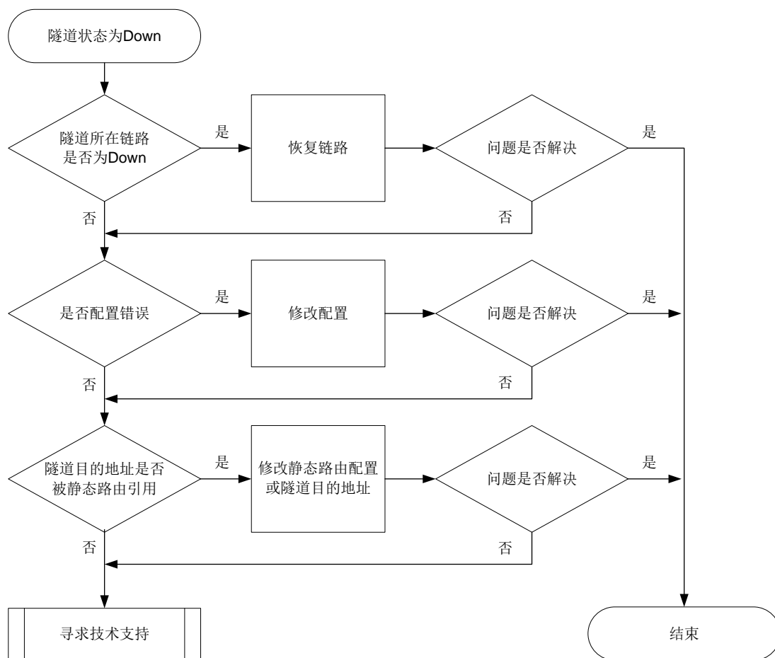
图10-16 MPLS TE 隧道状态为 Down 的故障诊断流程图
