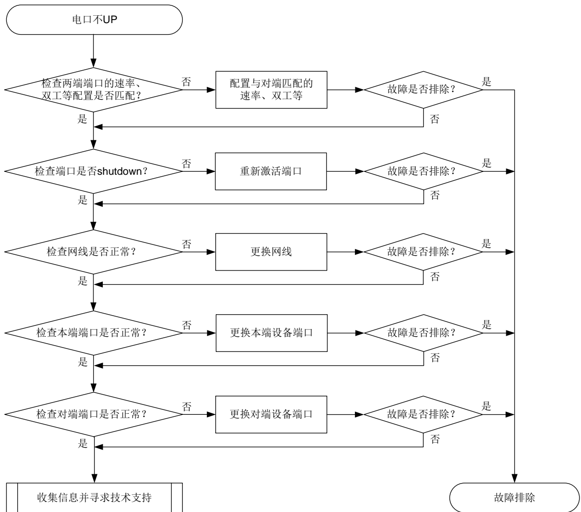
图2-19 故障诊断流程图
