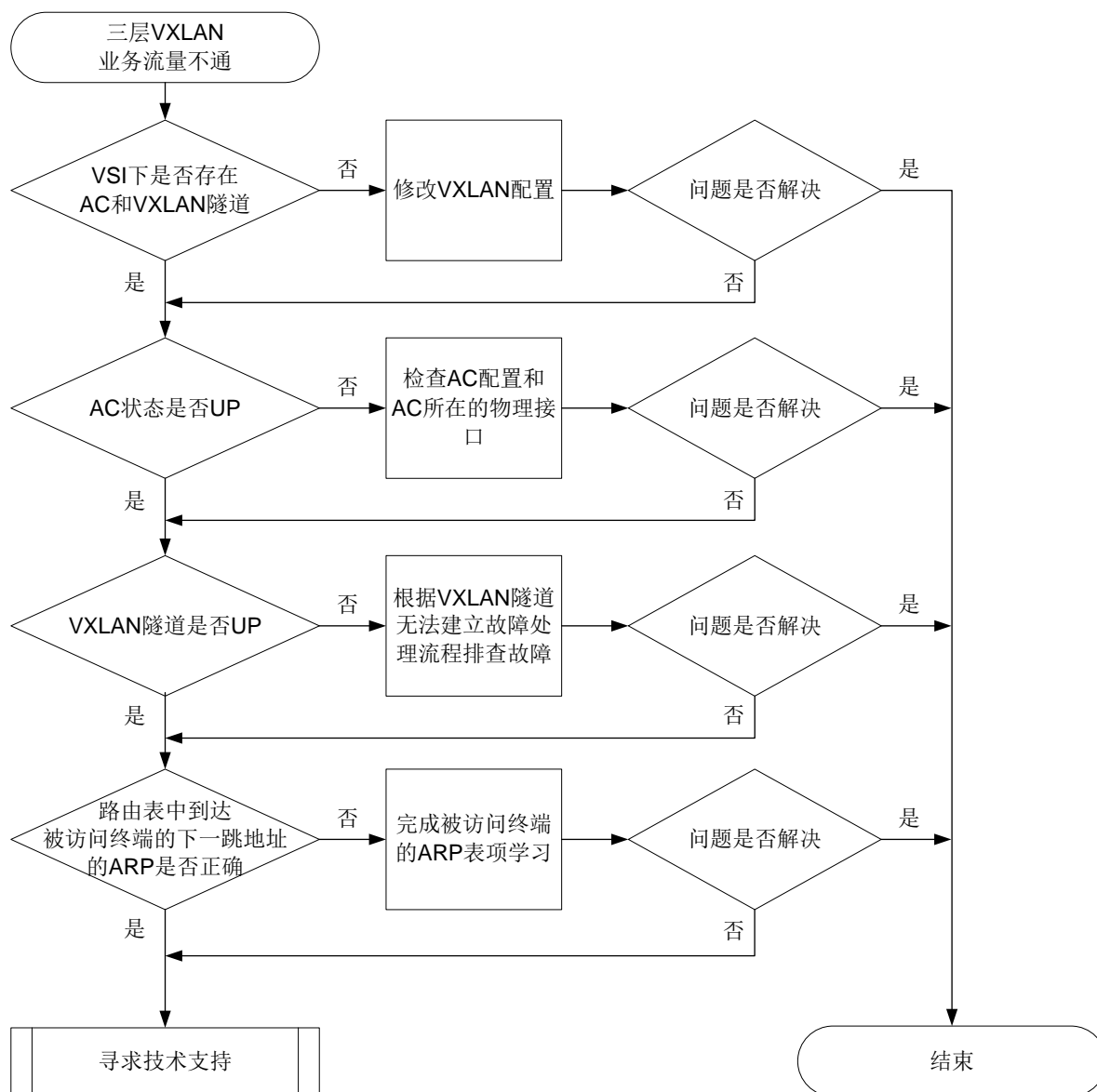
图13-4 三层 VXLAN 业务流量不通的故障诊断流程图
