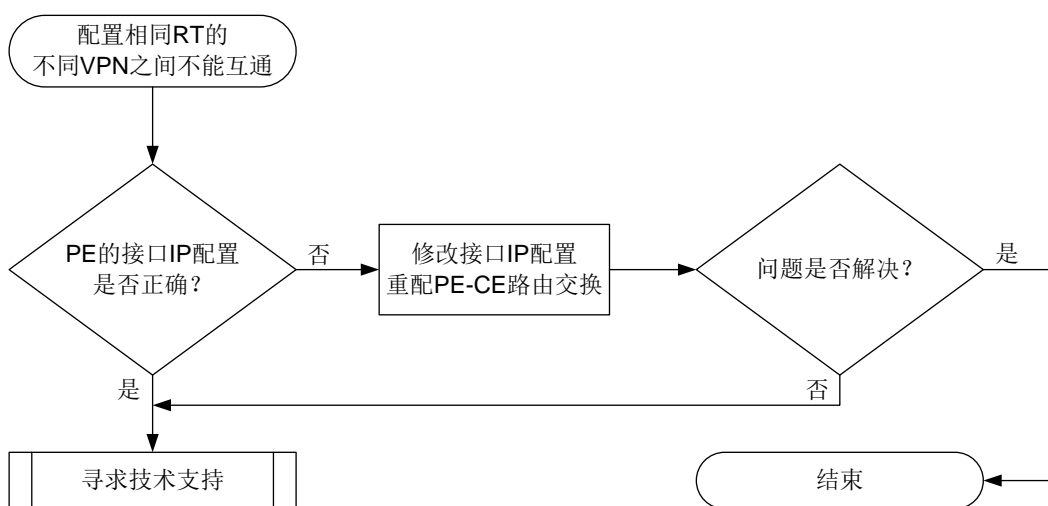
图10-10 配置相同 RT 的不同 VPN 之间不能互通的故障诊断流程图
