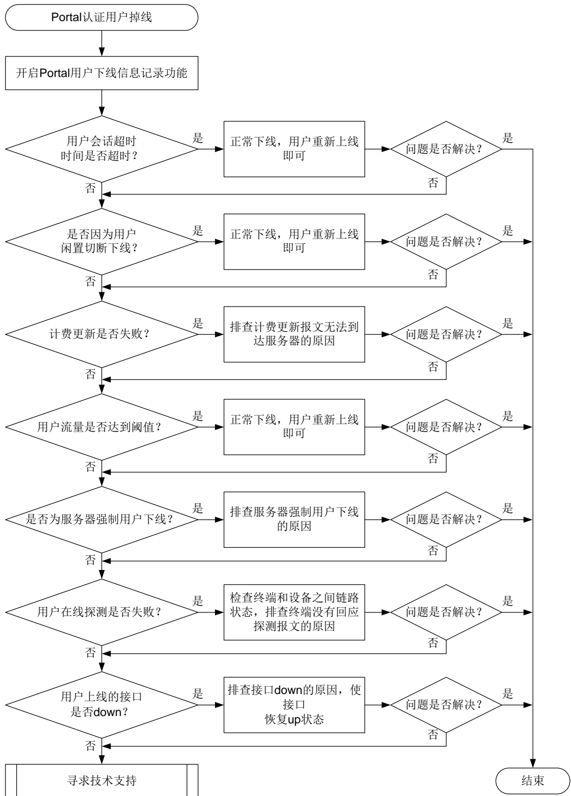
图15-27 Portal认证用户掉线的故障诊断流程图
