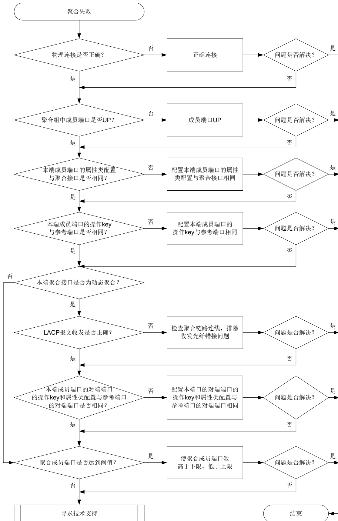
图6-6 聚合成员端口无法选中的故障诊断流程图
