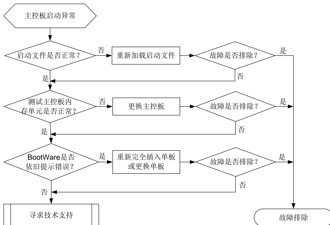
图2-12 故障诊断流程图
