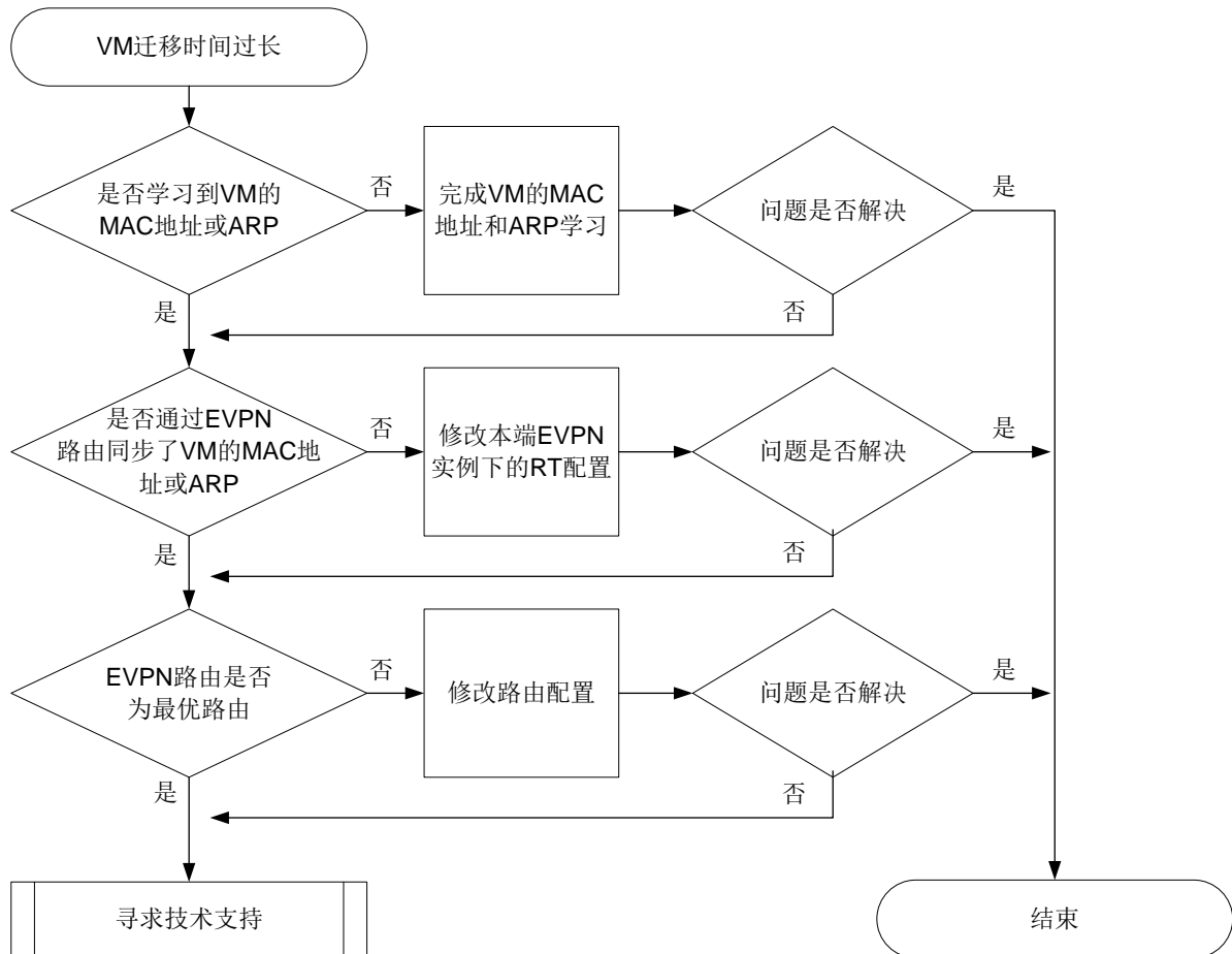
图13-5 VM 迁移时间过长的故障诊断流程图
