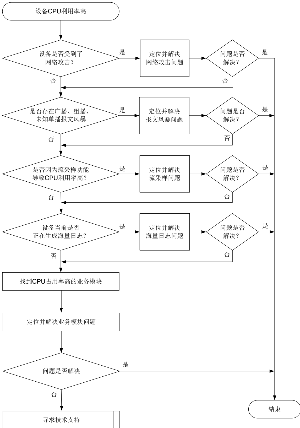
图4-1 CPU 占用率高的故障诊断流程图
