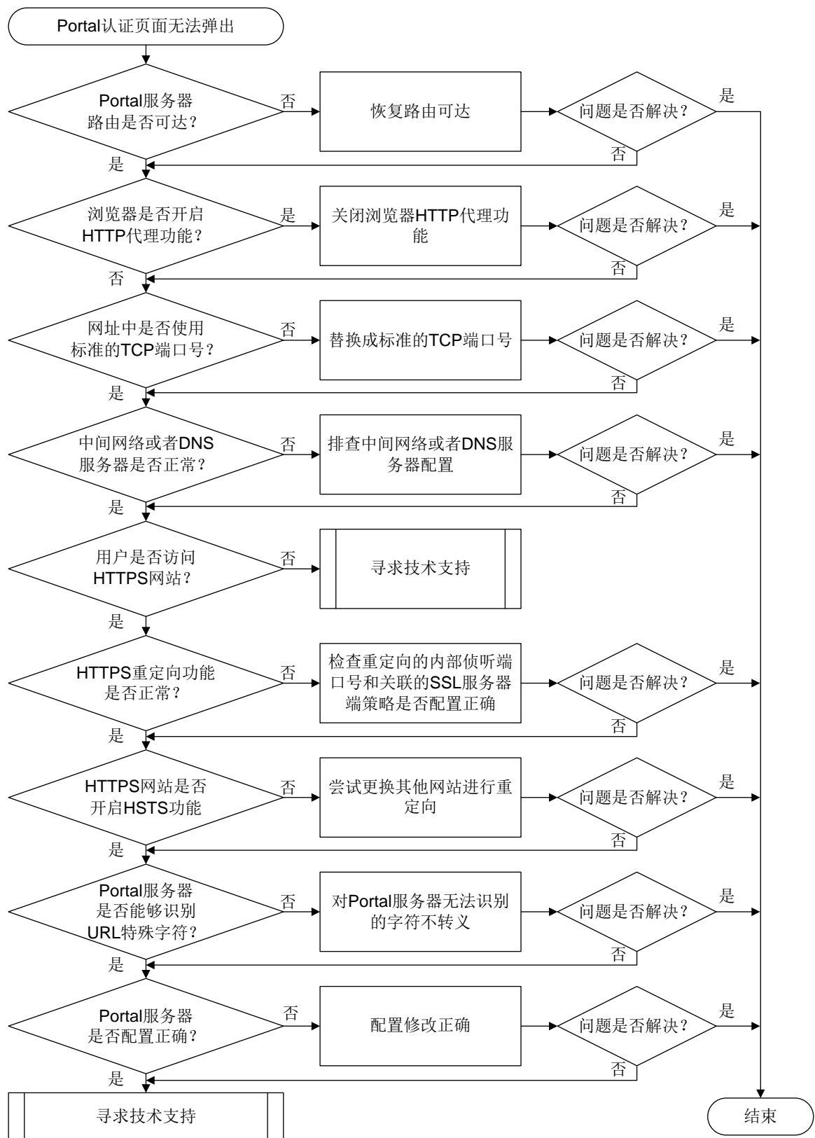
图15-21 Portal 认证页面无法弹出的故障诊断流程图
