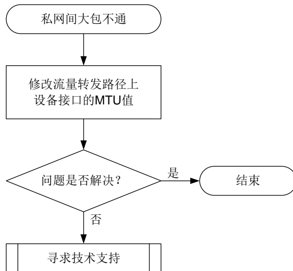
图10-13 私网间大包不通故障诊断流程图
