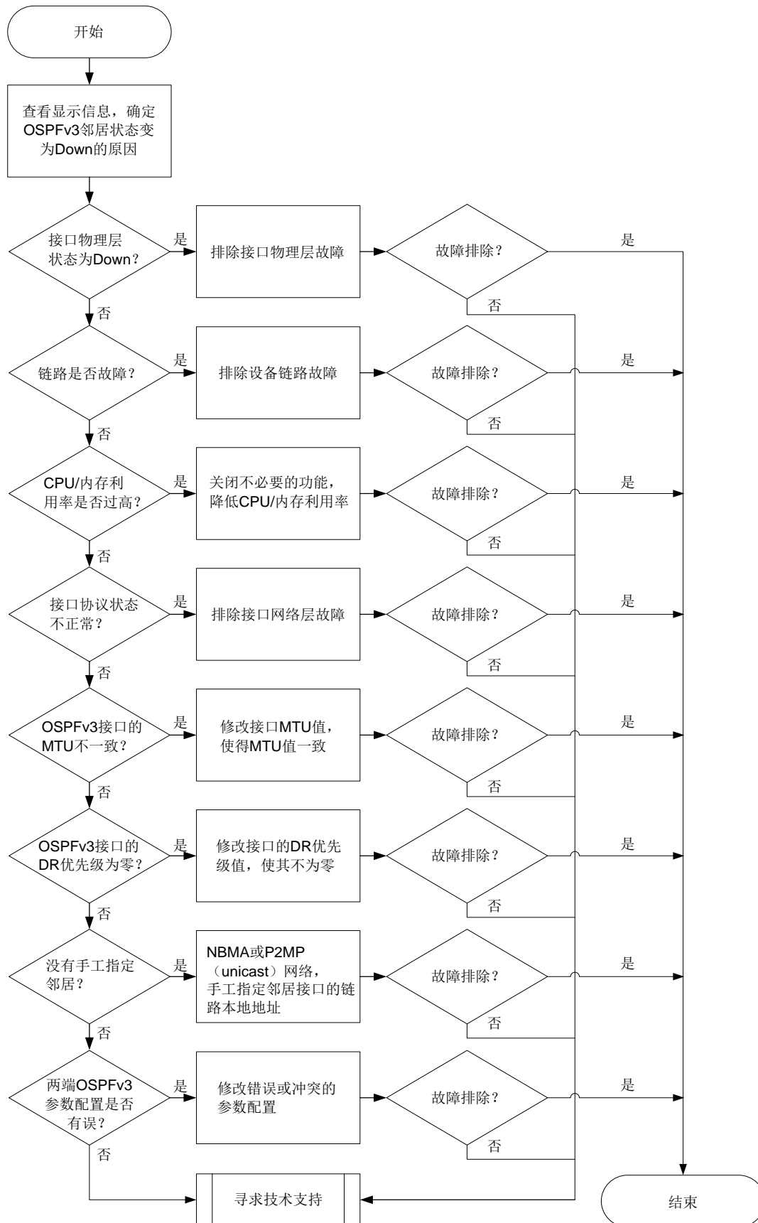
图8-6 OSPFv3 邻居 Down 的故障诊断流程图
