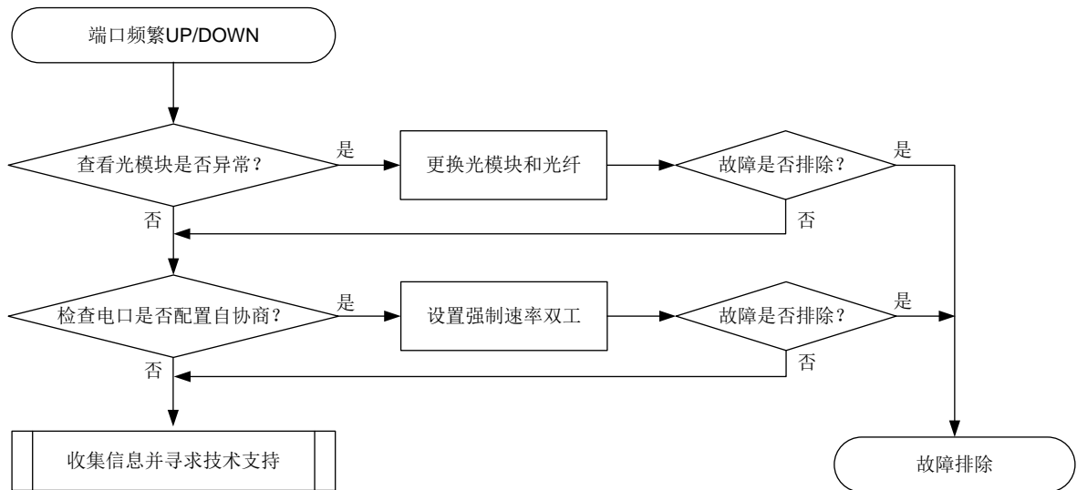
图2-20 故障诊断流程图
