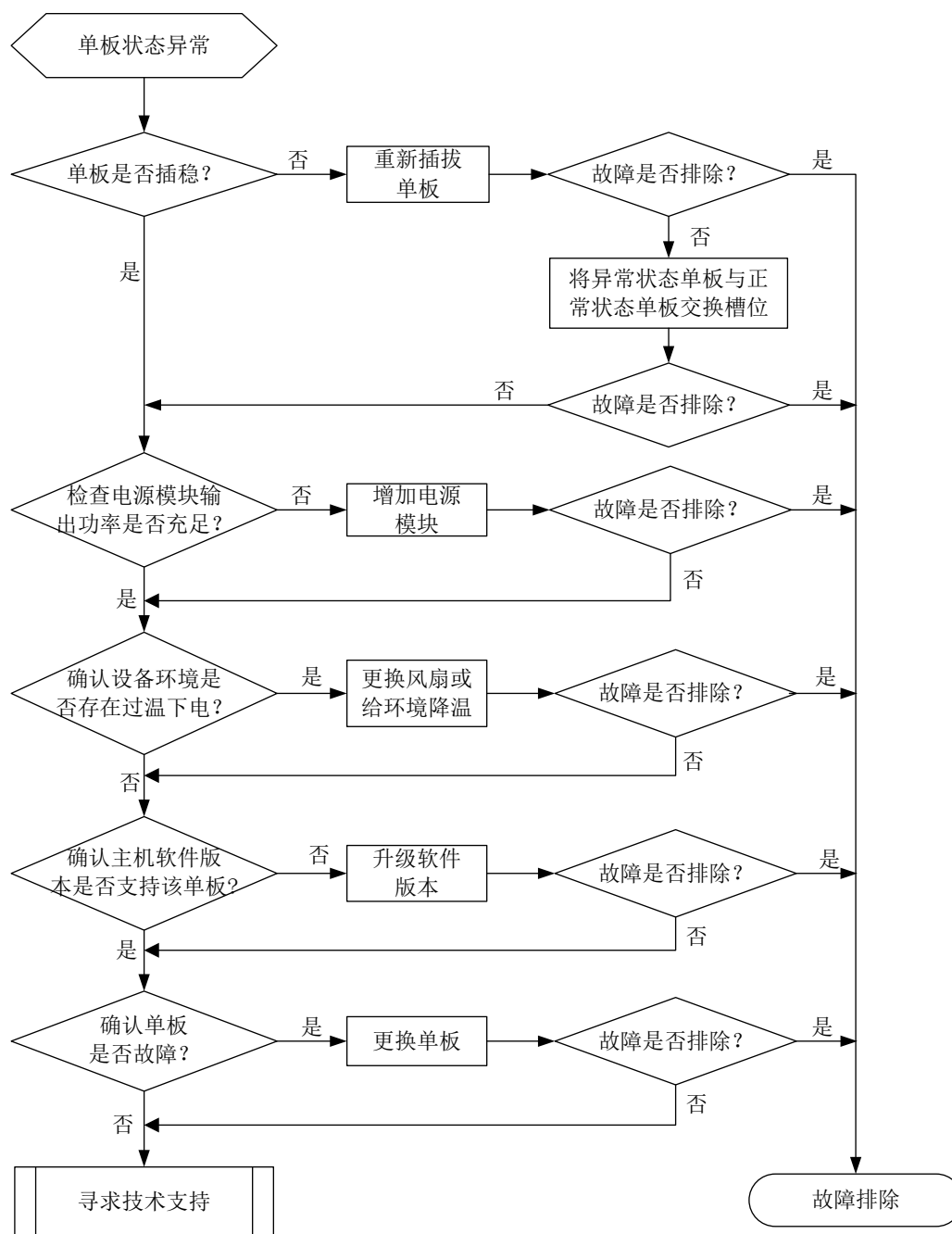
图2-9 单板状态异常故障诊断流程图
