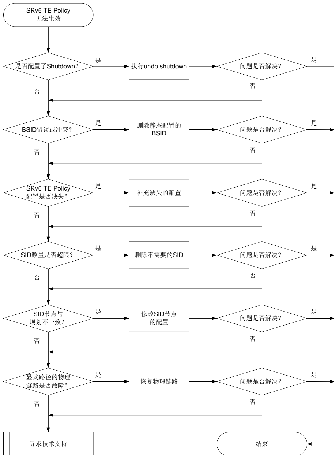
图11-5 SRv6 TE Policy 无法生效的故障诊断流程图
