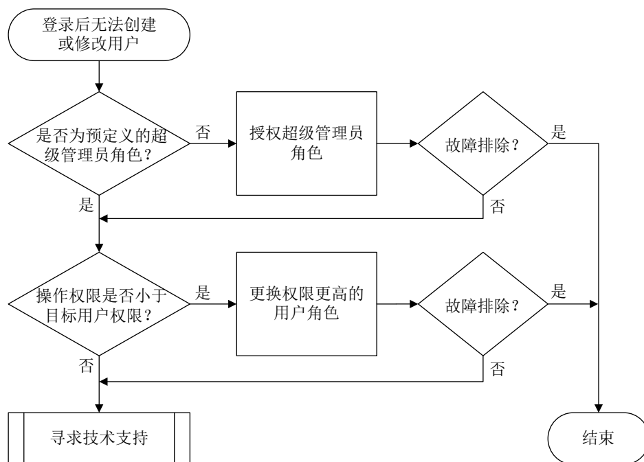
图15-2 登录后无法创建或修改本地用户的故障诊断流程图
