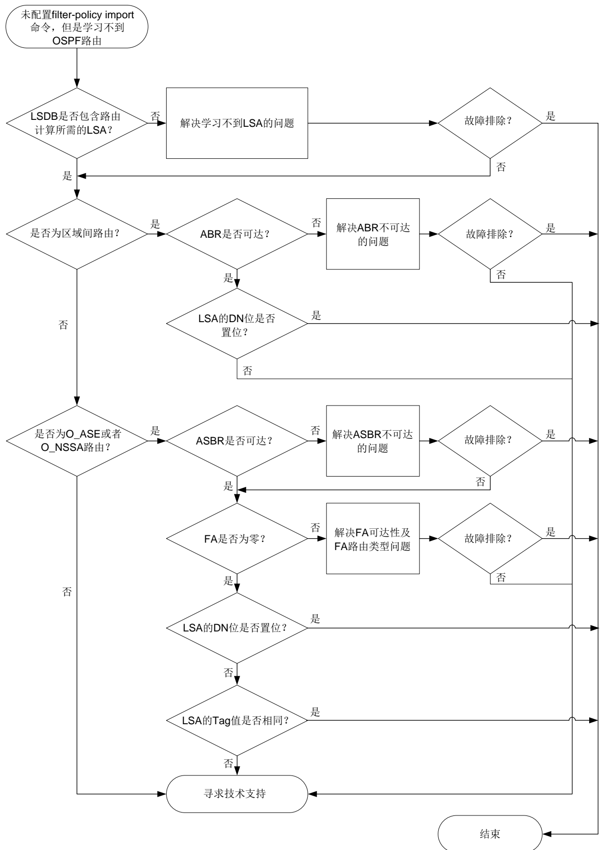
图8-11 设备学习不到 OSPF 路由故障诊断流程图二
