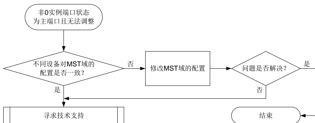
图6-3 非 0 实例端口状态为主端口且无法调整的故障处理流程图
