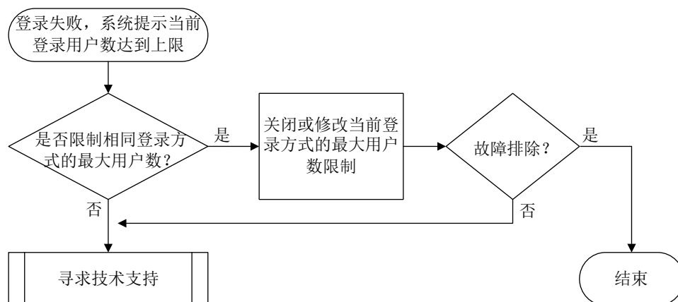
图15-10 使用相同登录方式接入用户数达到上限后的故障诊断流程图
