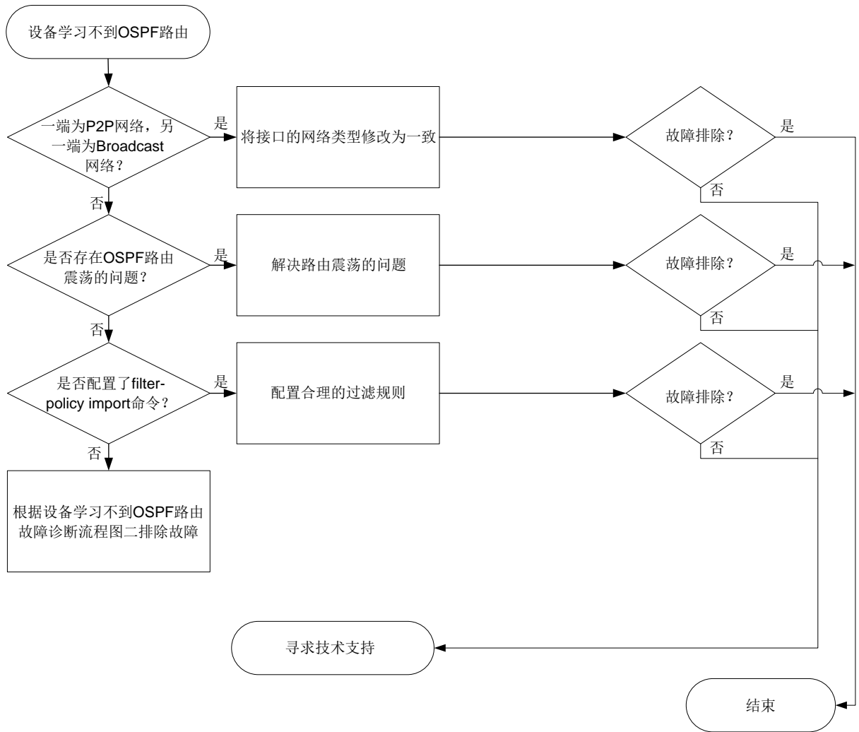
图8-10 设备学习不到 OSPF 路由故障诊断流程图一
