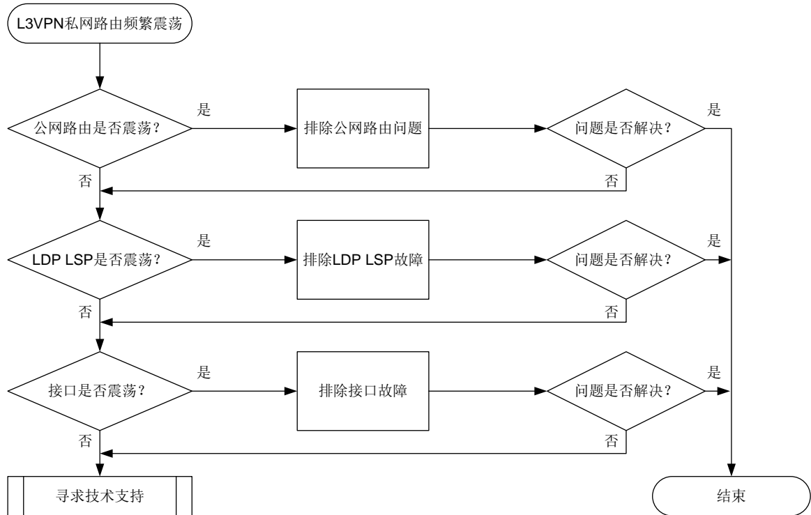
图10-7 L3VPN私网路由频繁震荡故障诊断流程图
