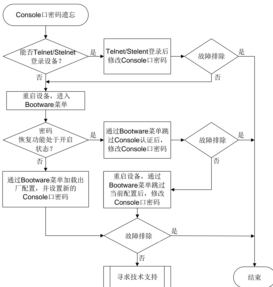
图3-1 Console 口密码遗忘故障诊断流程图
