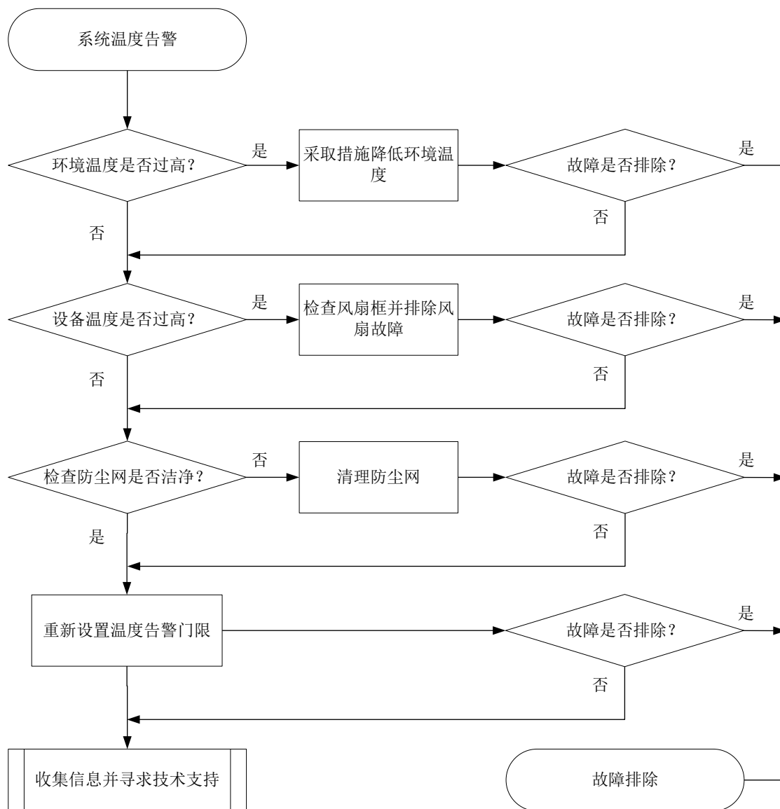
图2-3 温度异常故障诊断流程图
