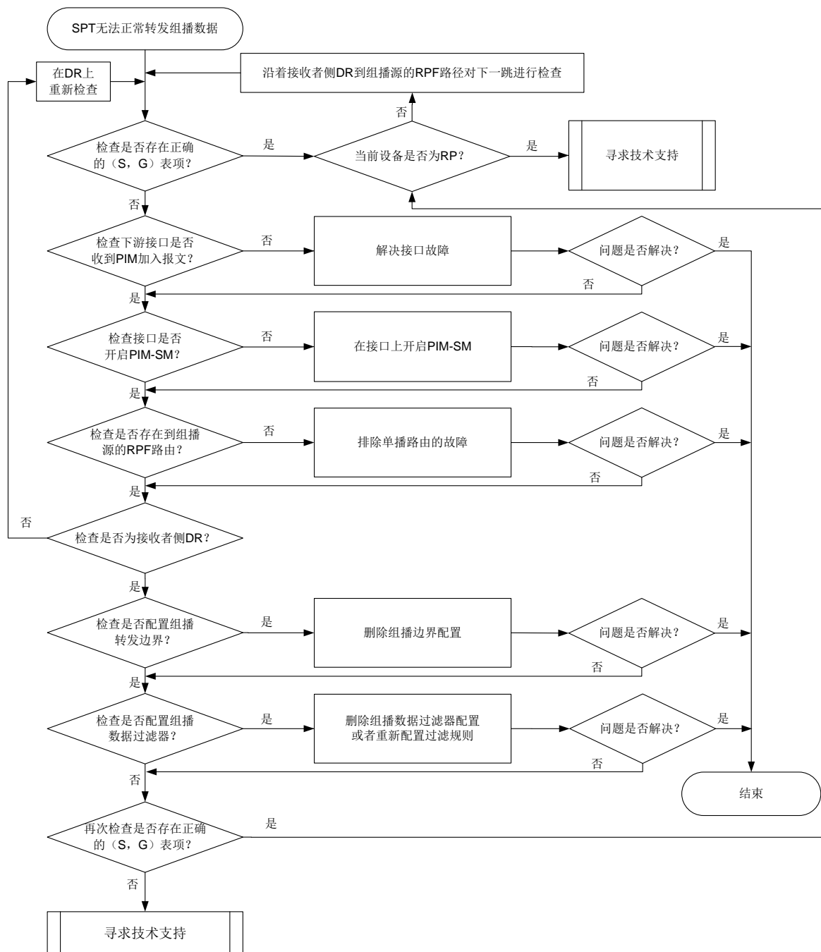
图9-4 PIM-SM 网络中 SPT 无法正常转发数据故障诊断流程图
