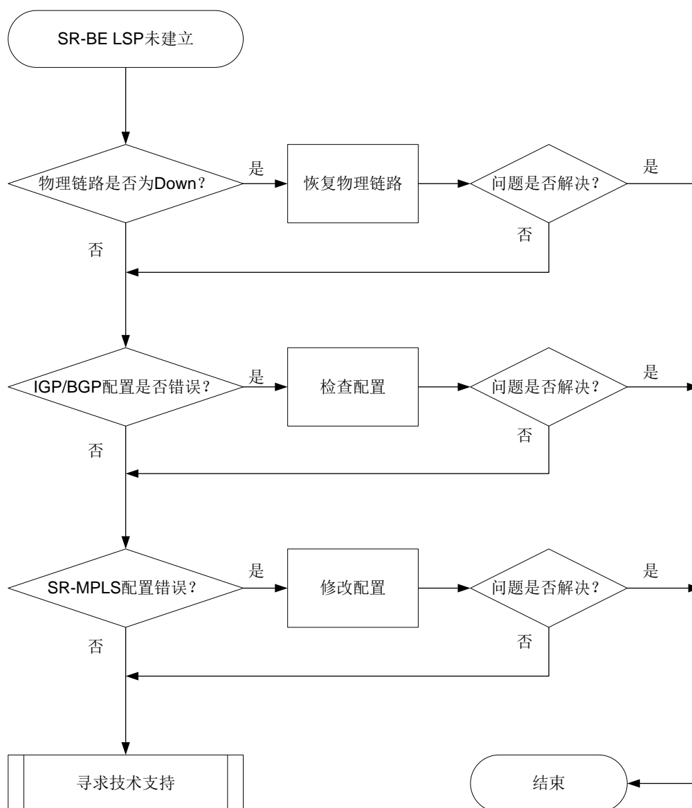
图11-3 采用 SR-BE 方式无法建立 SRLSP 的故障诊断流程图
