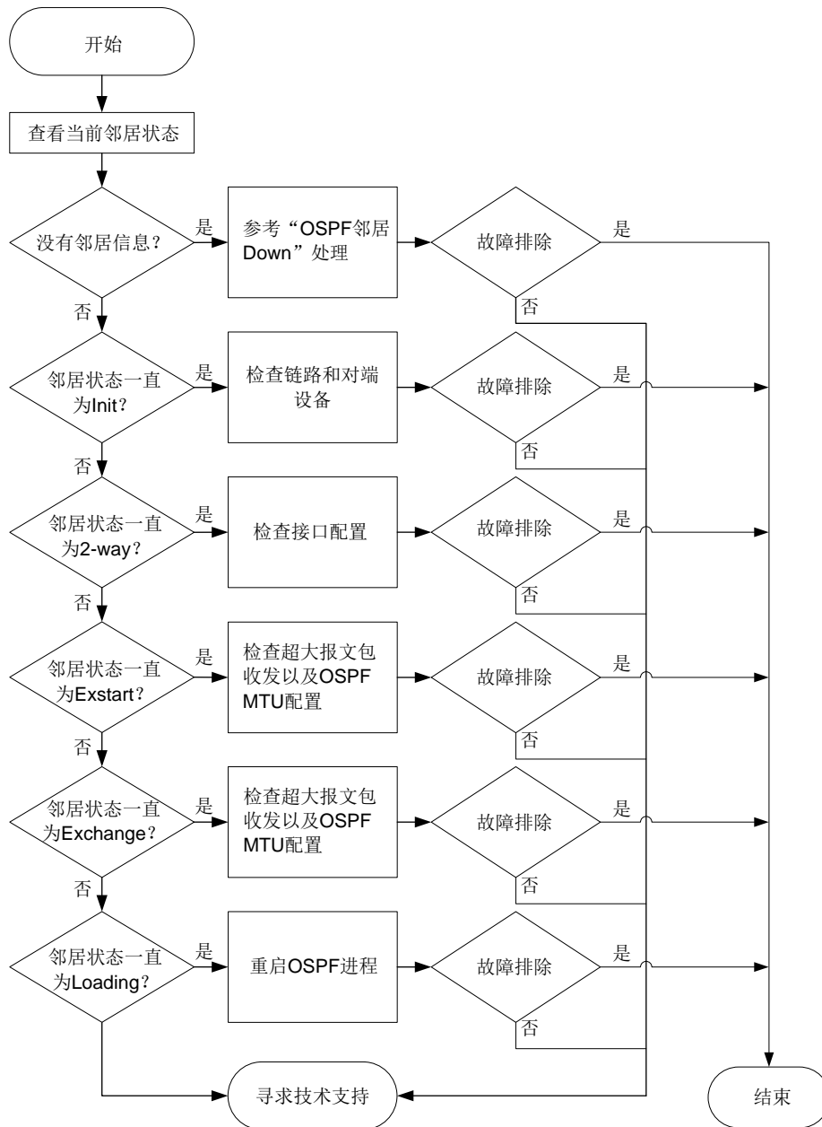
图8-9 OSPF 邻居无法达到 FULL 状态的故障诊断流程图
