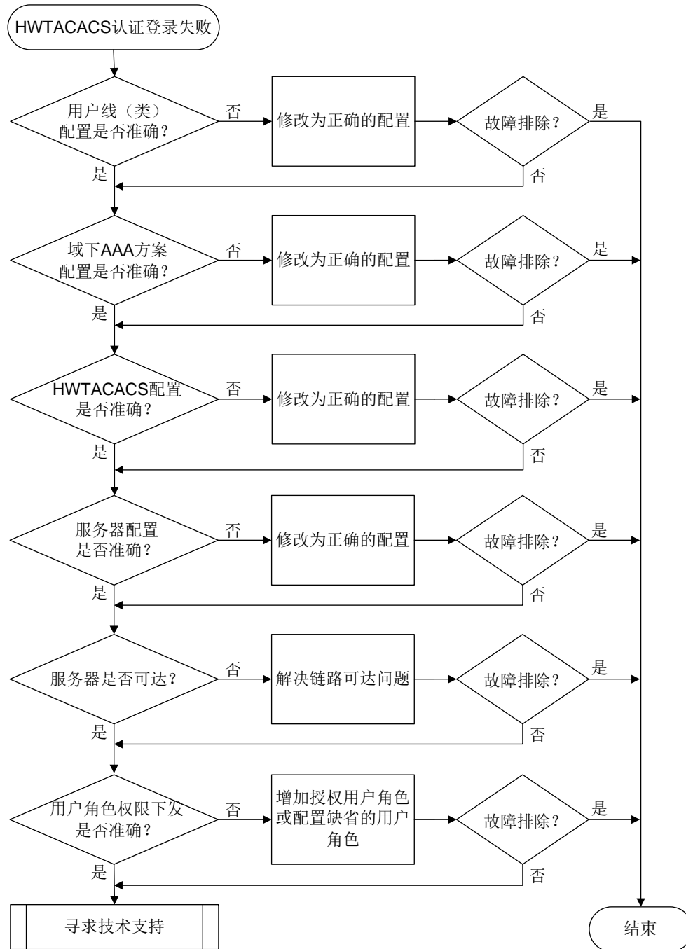
图15-16 HWTACACS 认证登录失败的故障诊断流程图
