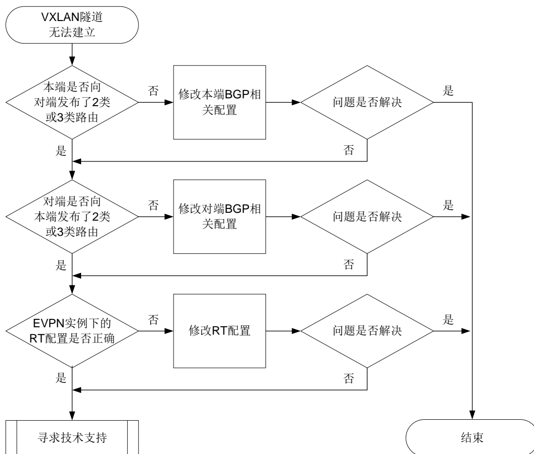
图13-1 同一 VXLAN 内 VTEP 之间的 VXLAN 隧道无法建立的故障诊断流程图
