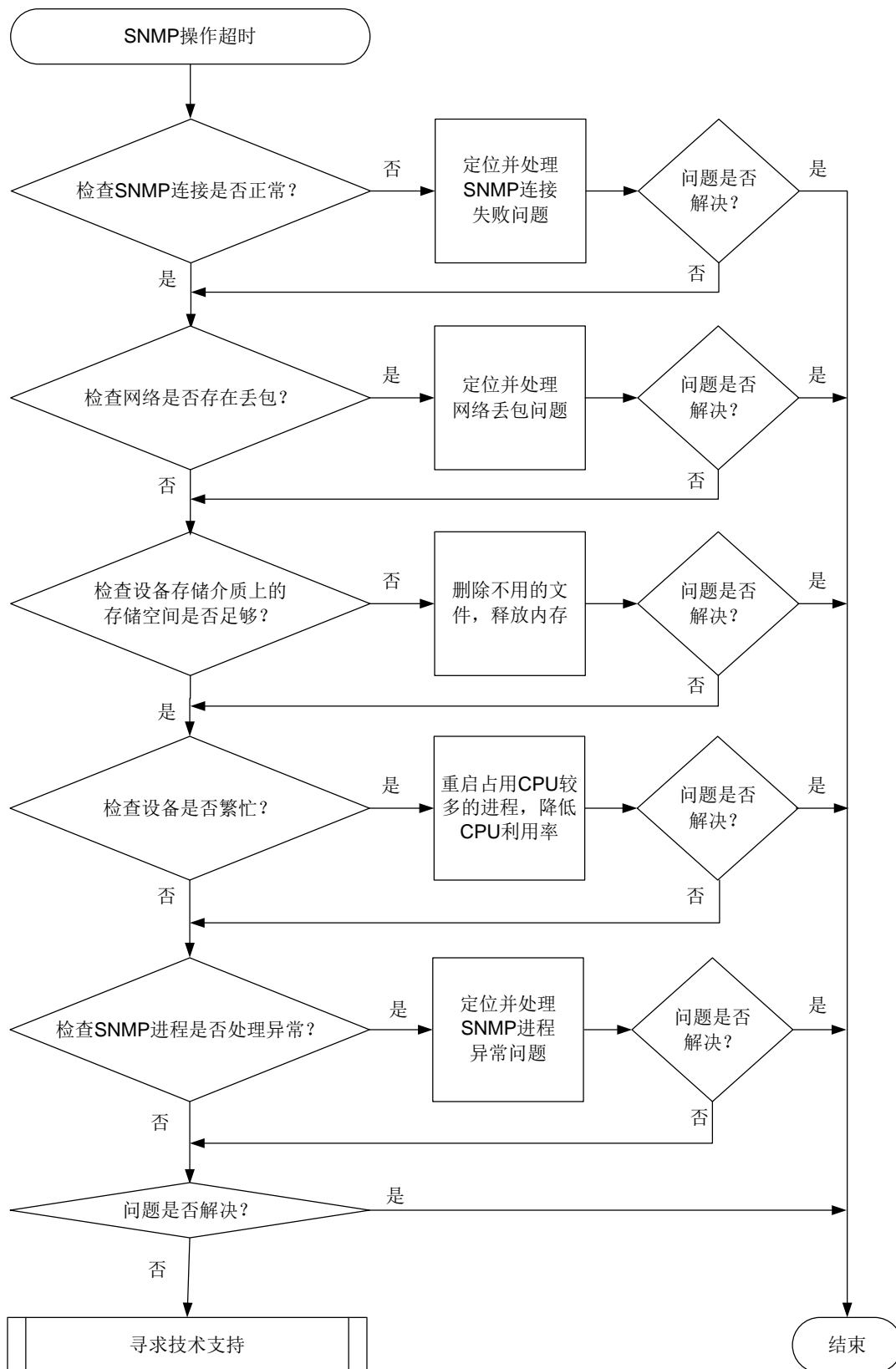
图18-4 SNMP 操作超时的故障诊断流程图
