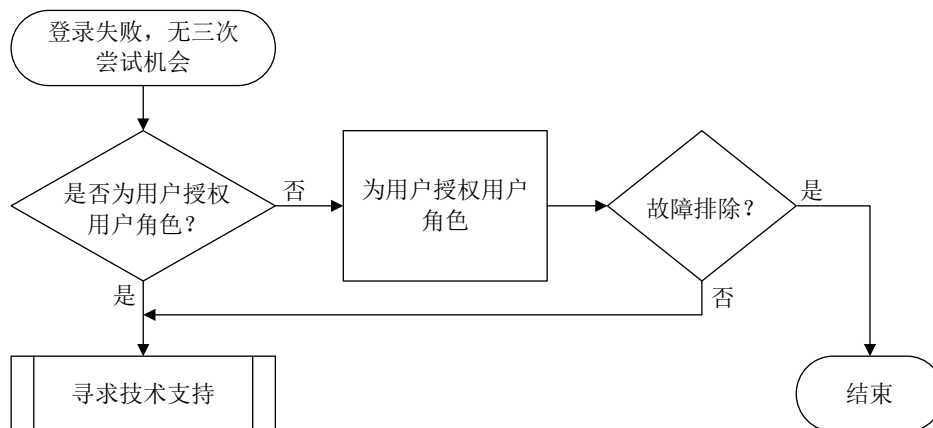
图15-3 管理员未被授权用户角色的故障诊断流程图
