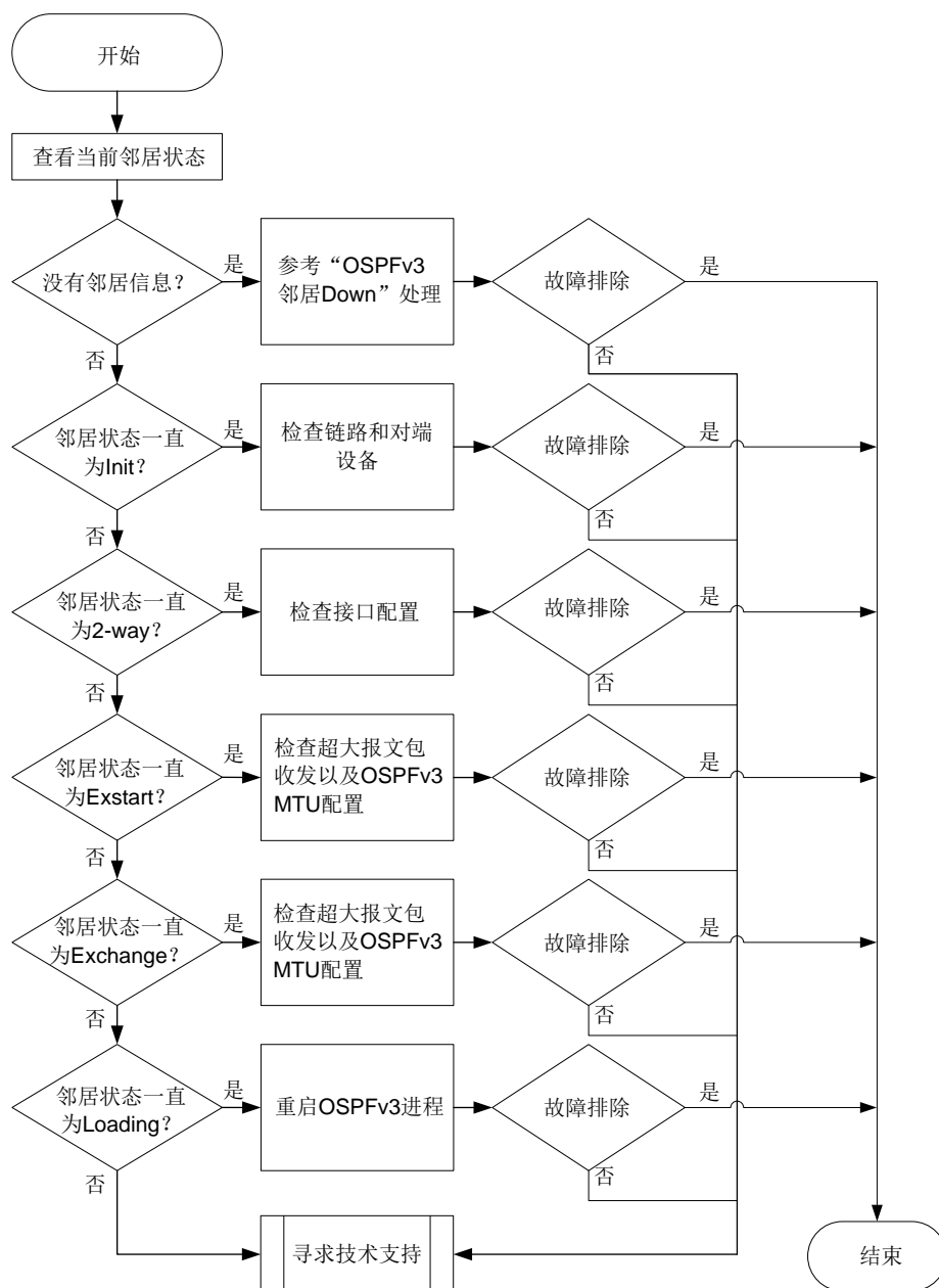
图8-7 OSPFv3 邻居 Down 的故障诊断流程图
