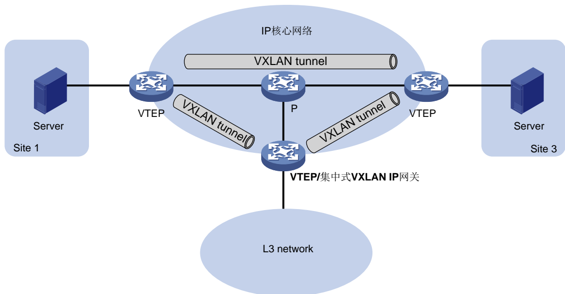
图12-1 集中式 VXLAN IP 网关示意图
