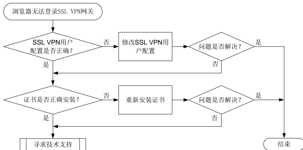
图16-4 浏览器无法登录 SSL VPN 网关的故障处理流程图
