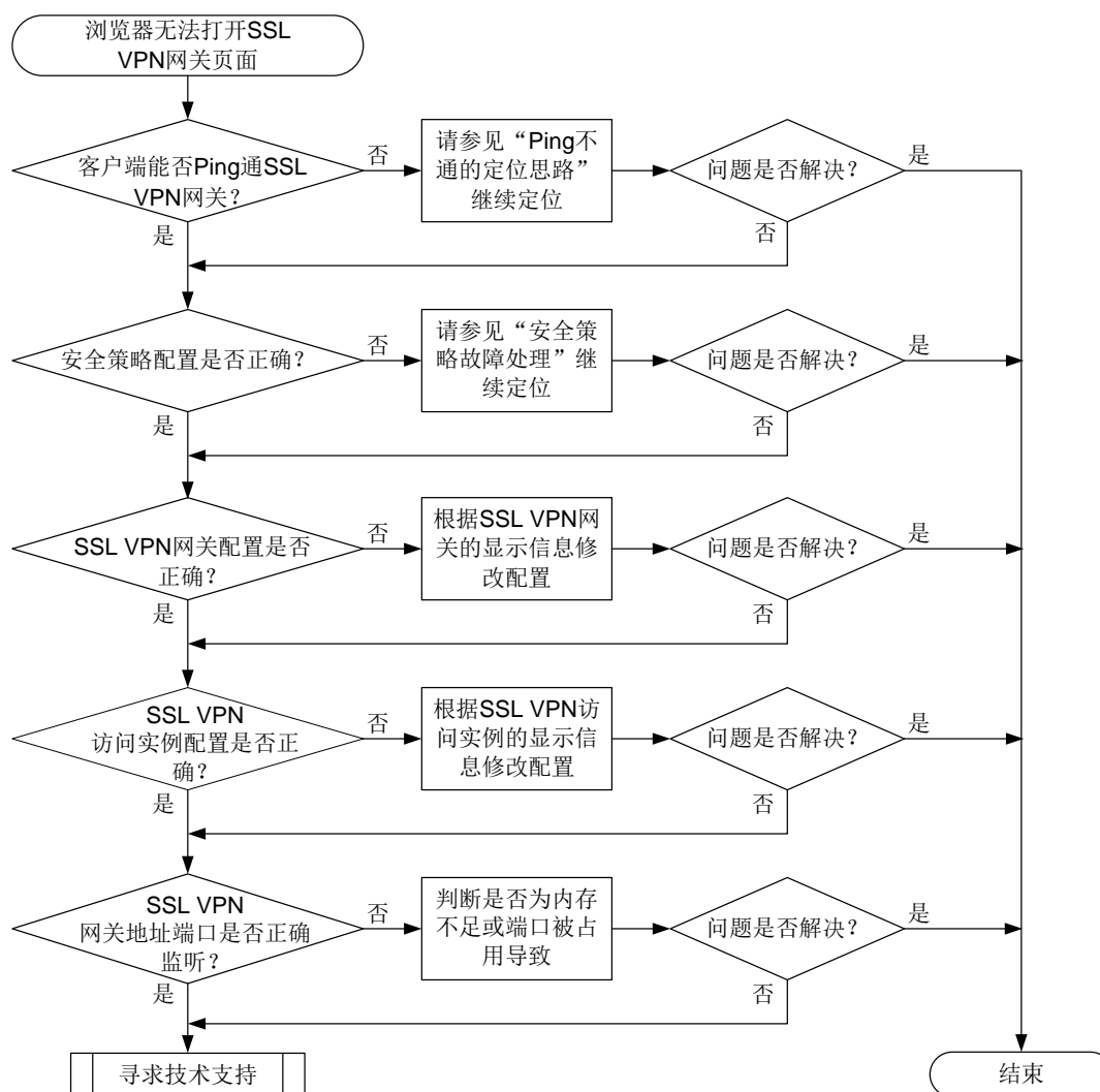
图16-2 浏览器无法打开 SSL VPN 网关页面的故障处理流程图
