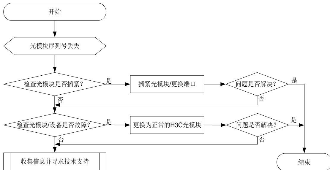
图2-24 故障诊断流程图
