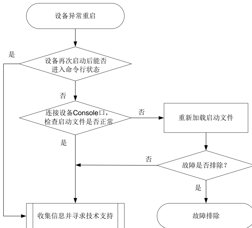
图2-2 设备异常重启故障诊断流程图
