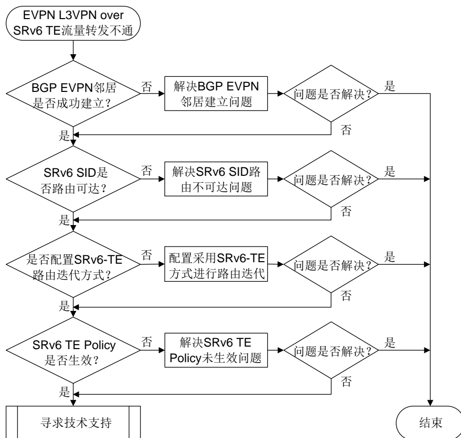
图11-2 EVPN L3VPN over SRv6 TE 流量转发不通的诊断流程图
