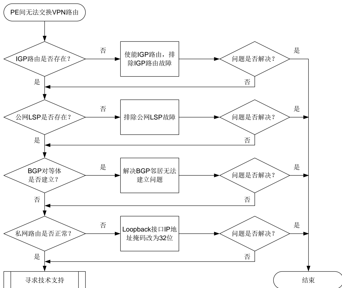
图10-8 PE 间无法交换私网路由故障诊断流程图
