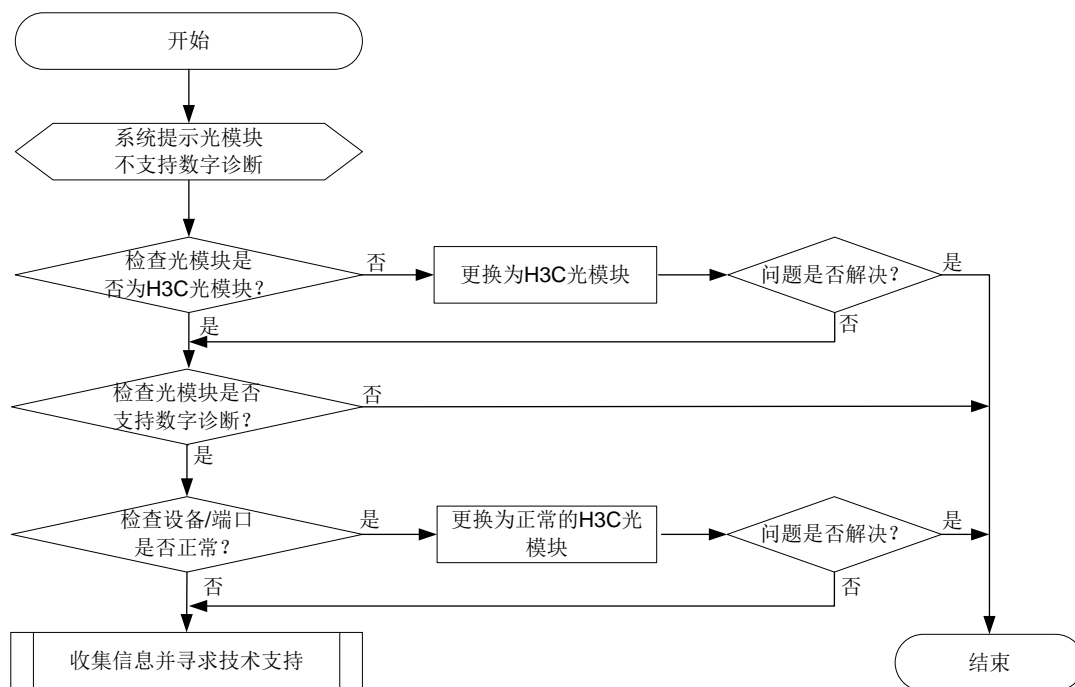
图2-23 故障诊断流程图
