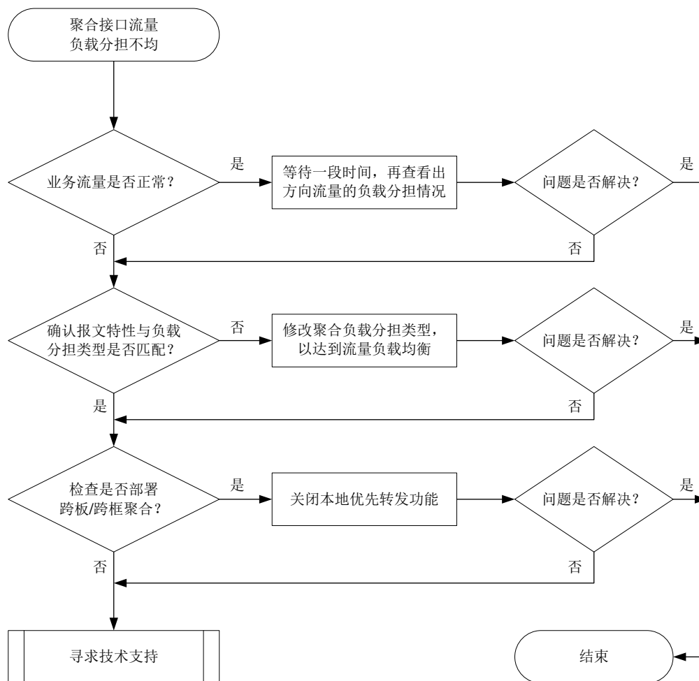
图6-5 聚合接口流量负载分担不均的故障诊断流程图
