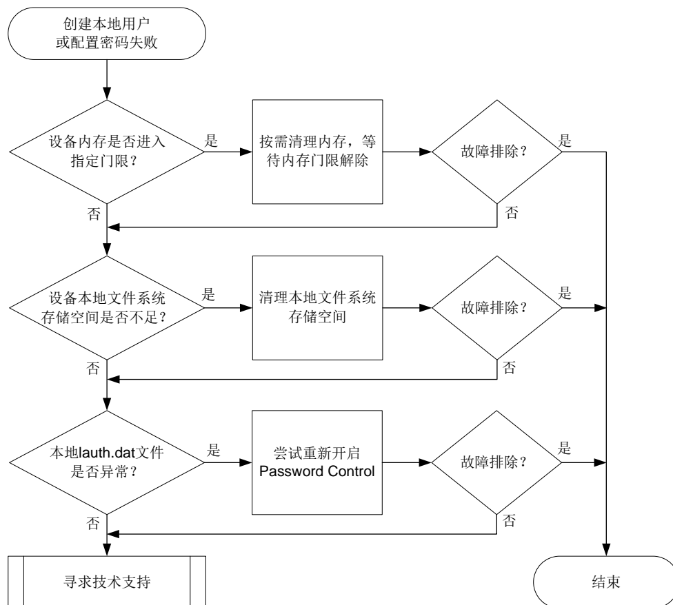
图15-19 创建本地用户或配置密码失败故障诊断流程图
