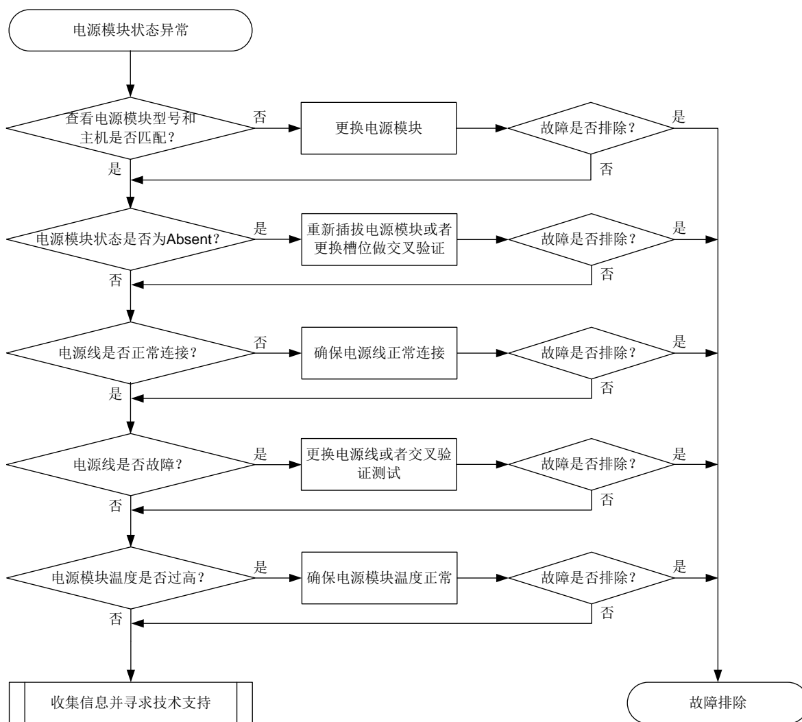
图2-7 故障诊断流程图
