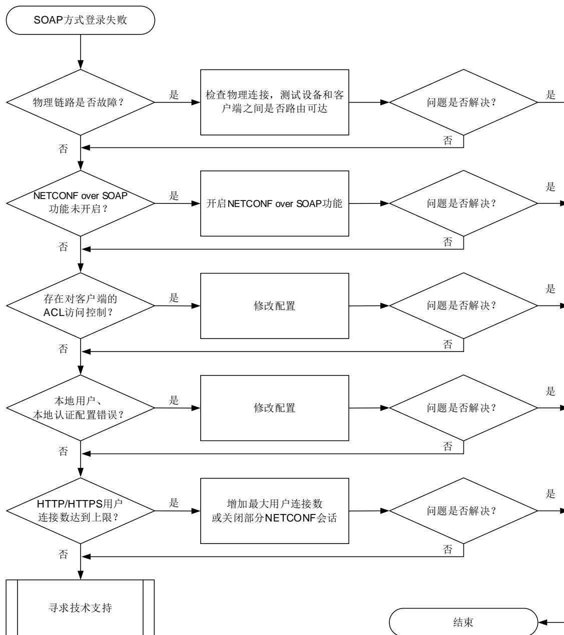
图17-1 SOAP 方式登录失败的故障诊断流程图
