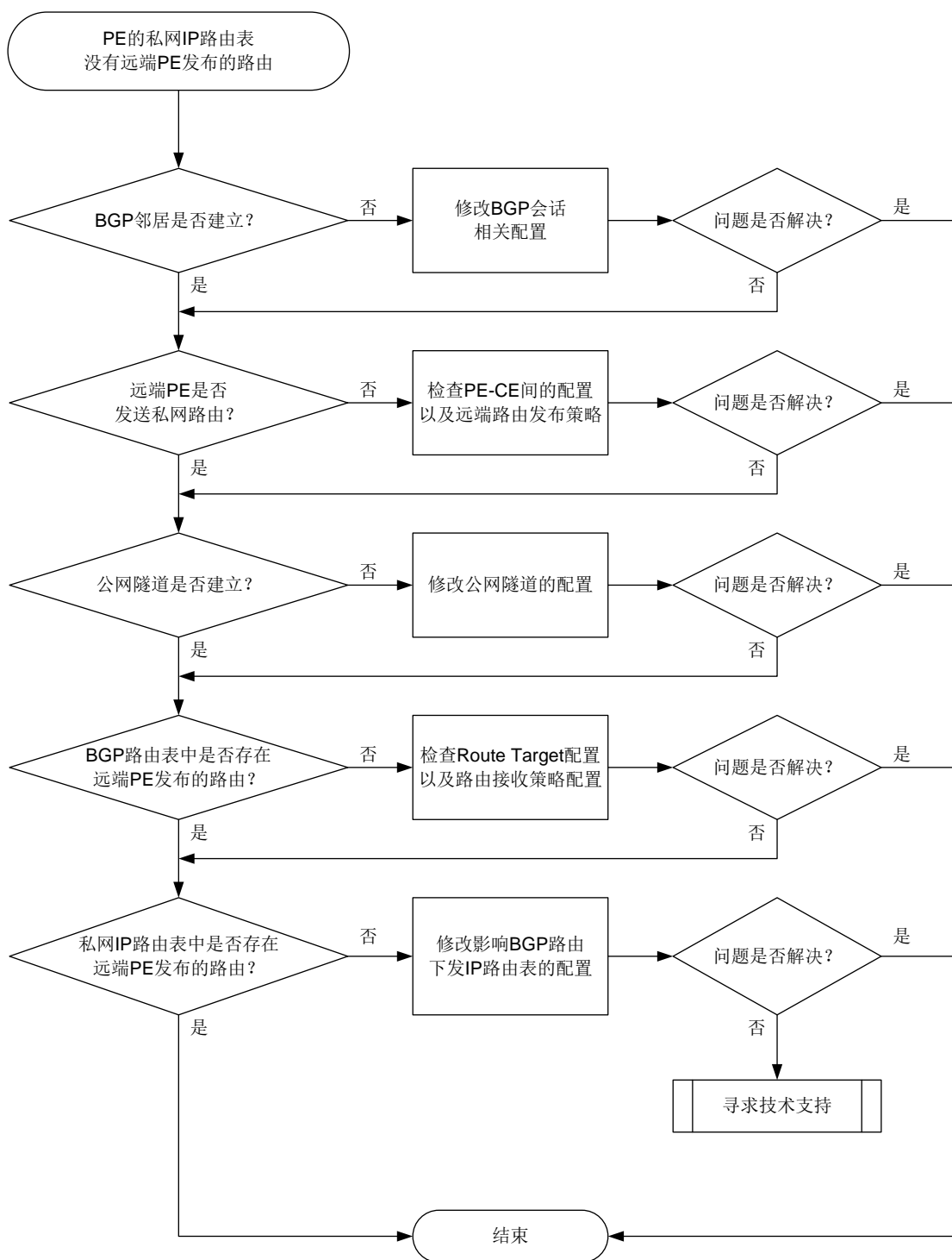
图10-12 PE 的私网 IP 路由表中没有远端 PE 发布的路由故障诊断流程图
