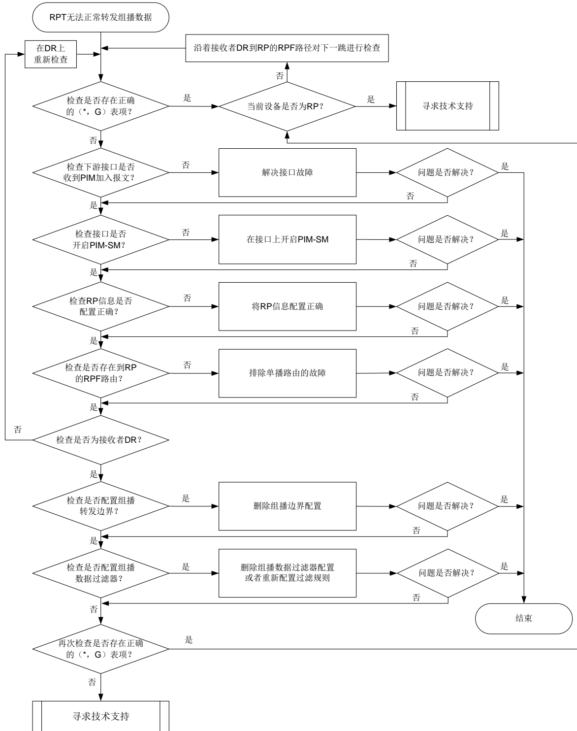
图9-5 PIM-SM 网络中 RPT 无法正常转发数据故障诊断流程图
