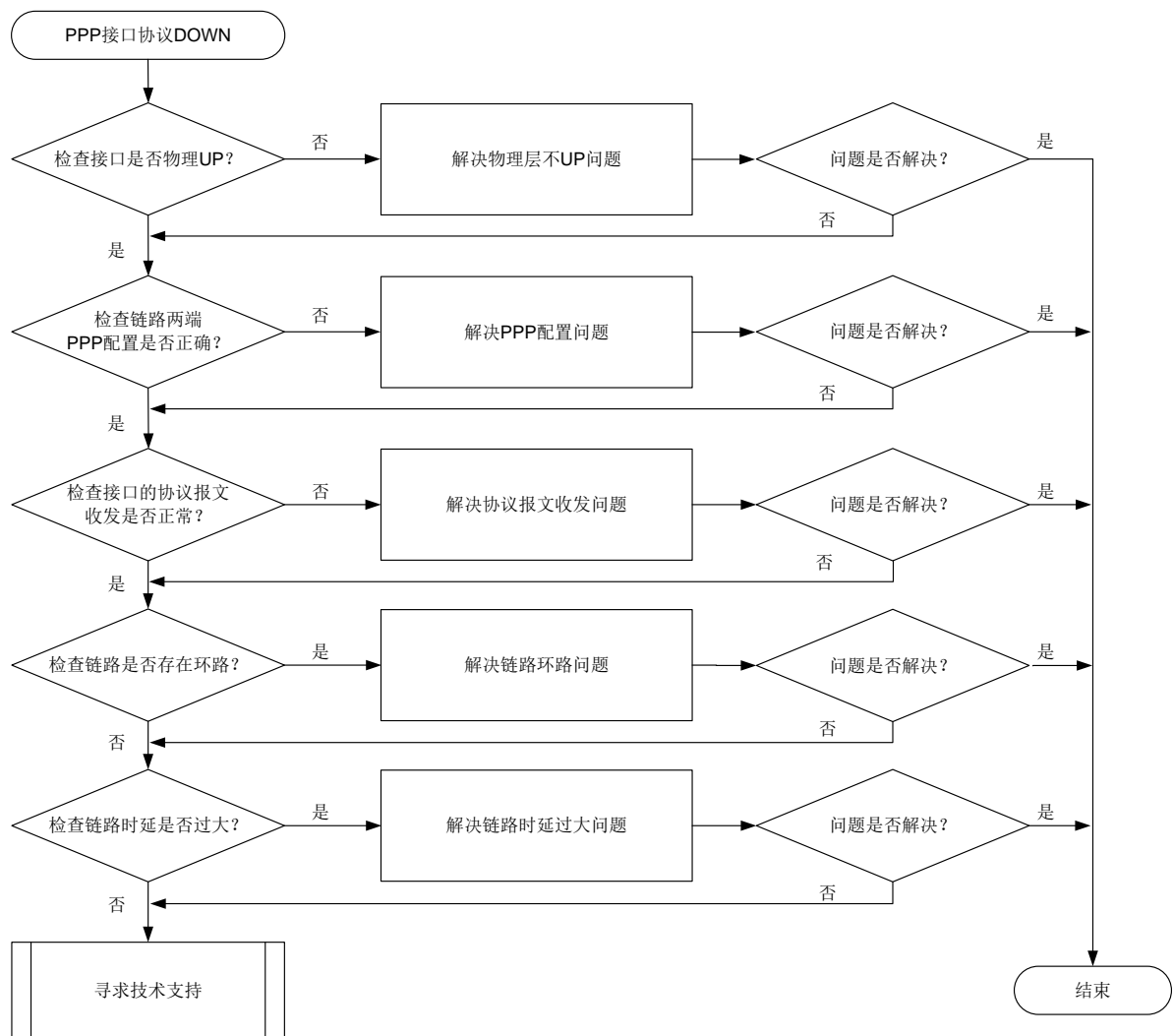
图7-1 PPP 接口协议 DOWN 的故障诊断流程图
