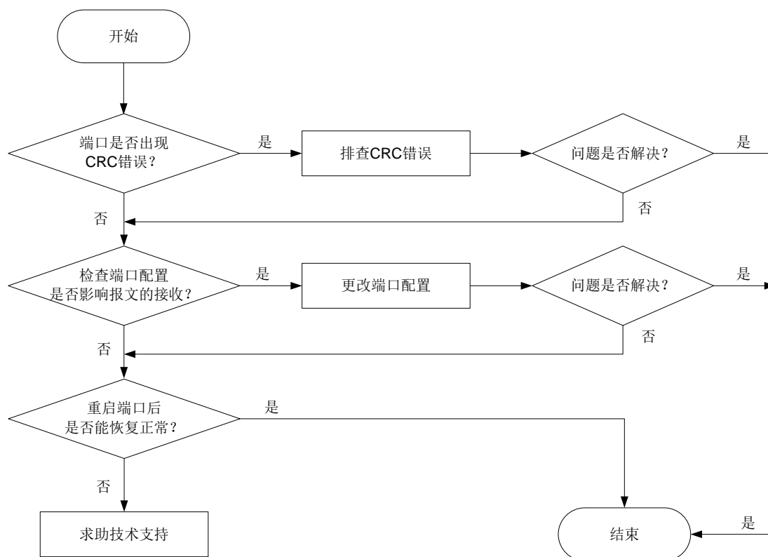
图2-17 故障诊断流程图
