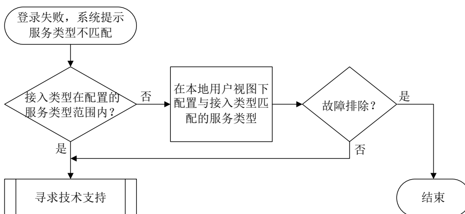
图15-6 本地用户服务类型不匹配的故障诊断流程图
