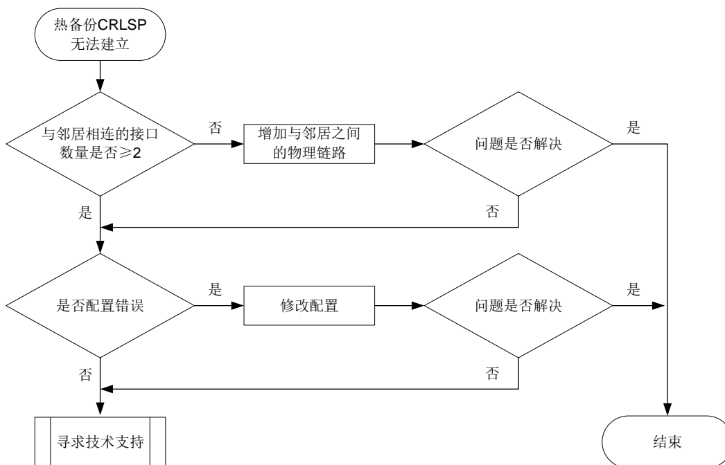
图10-19 热备份 CRLSP 无法建立的故障诊断流程图
