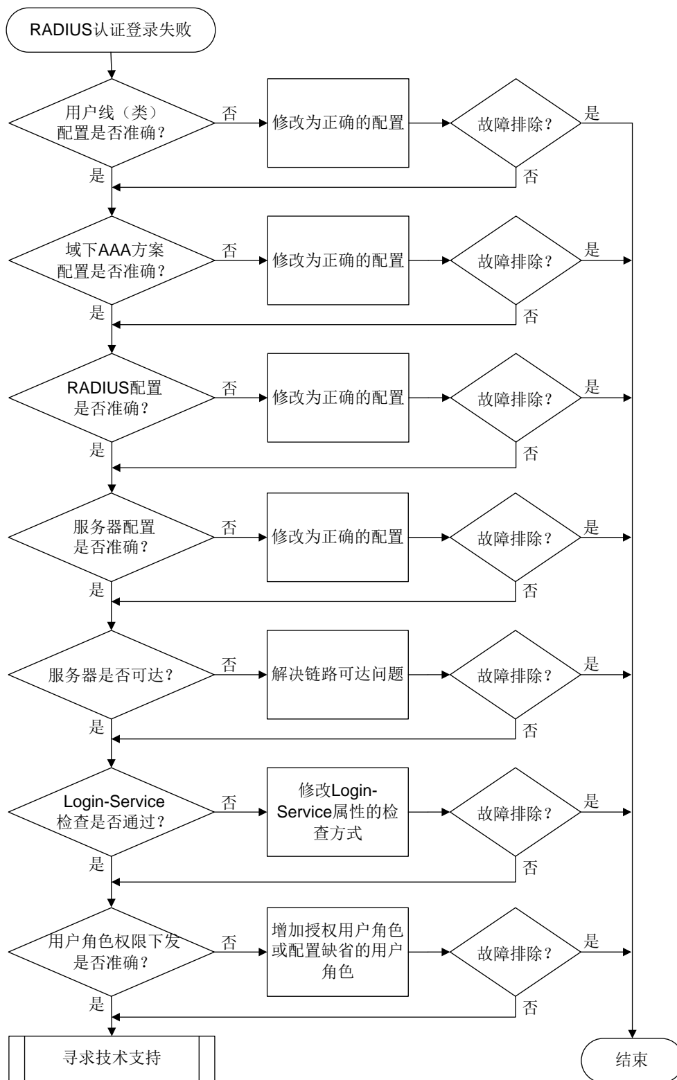
图15-15 RADIUS 认证登录失败的故障诊断流程图
