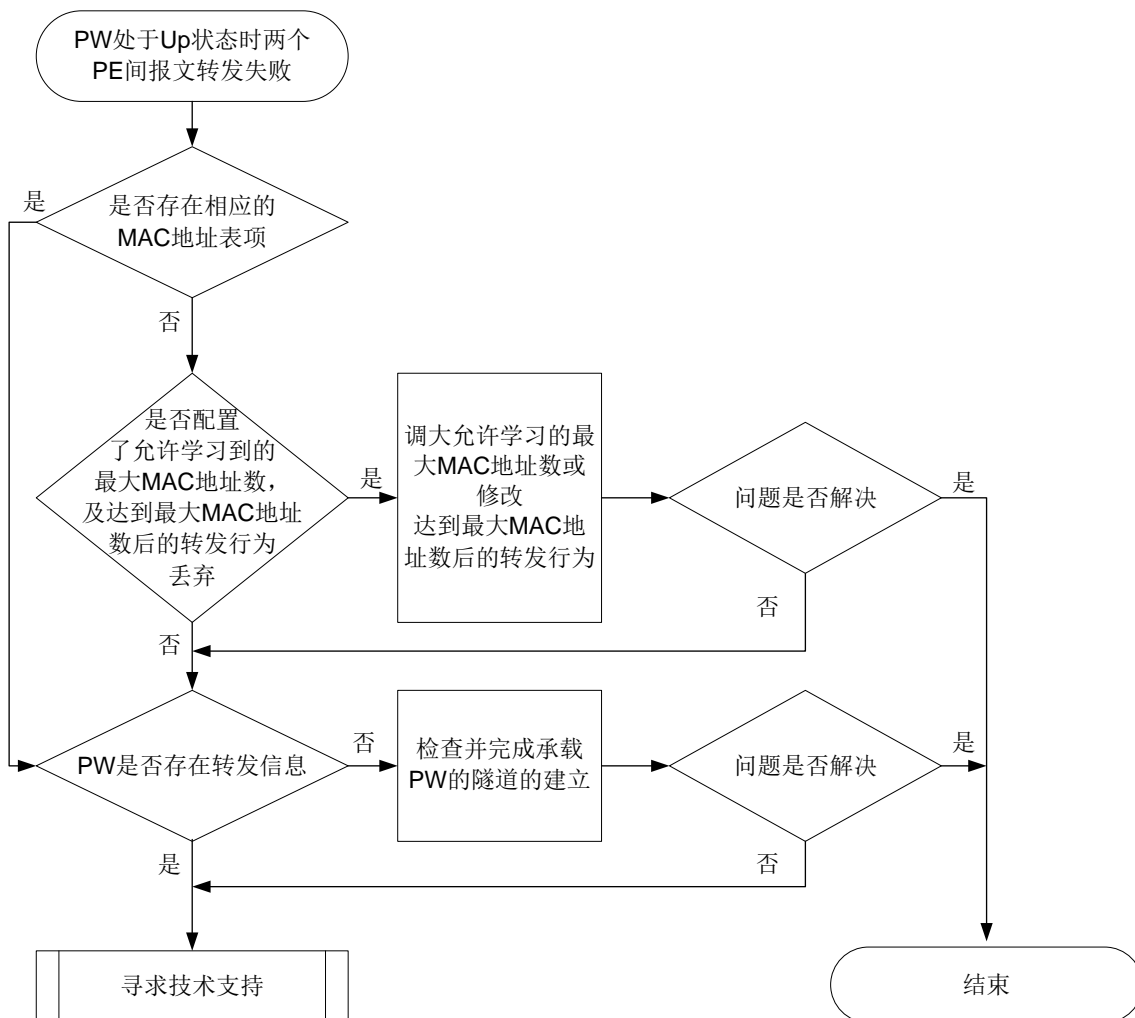
图10-22 PW 处于 Up 状态时两个 PE 间报文转发失败故障诊断流程图
