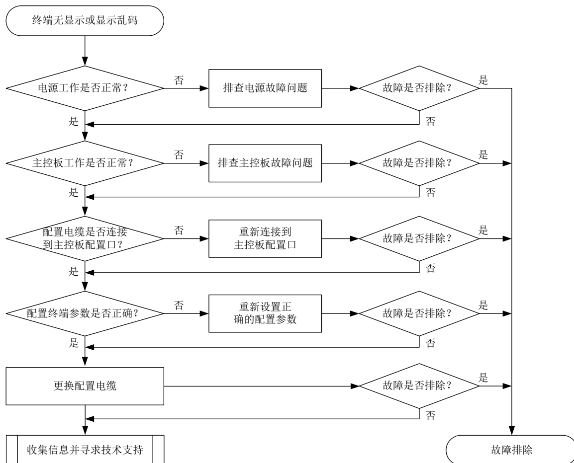
图2-1 故障诊断流程图
