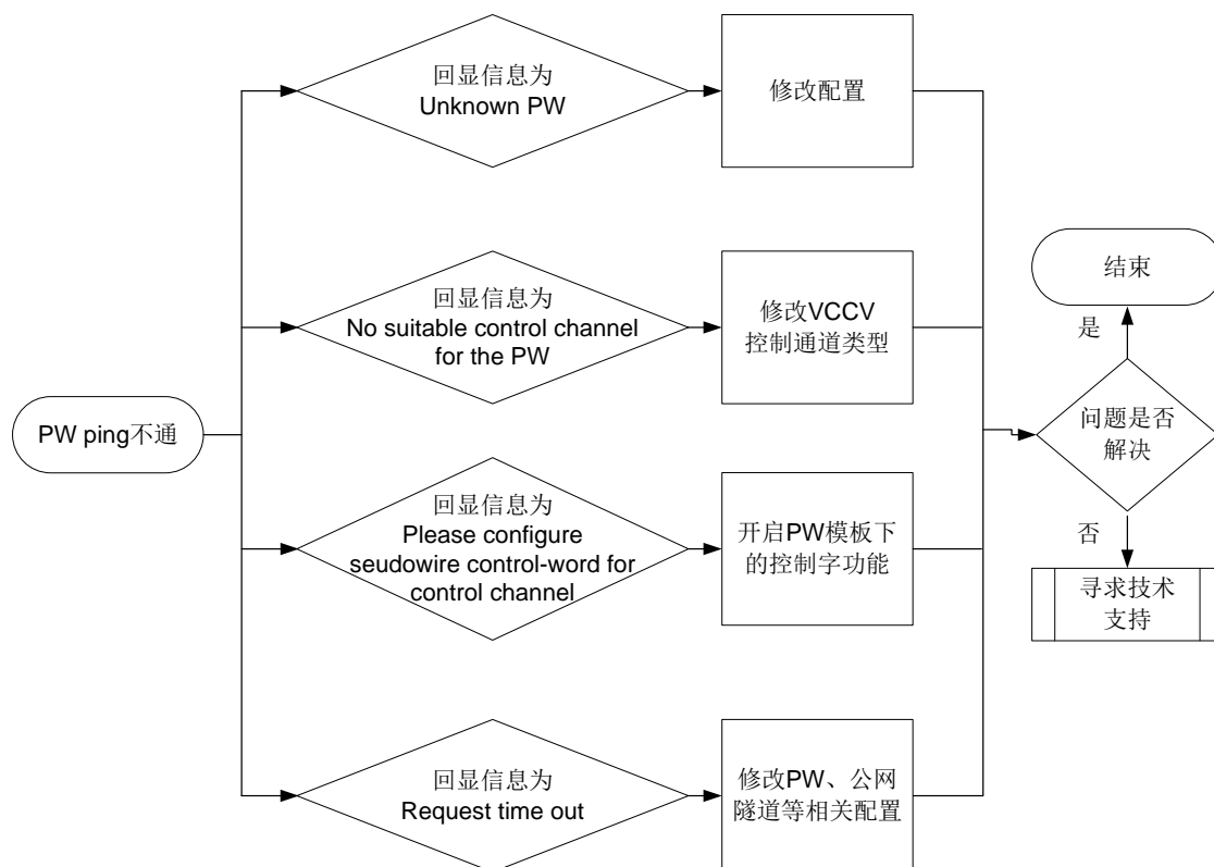
图10-5 PW ping 不通的故障诊断流程图
