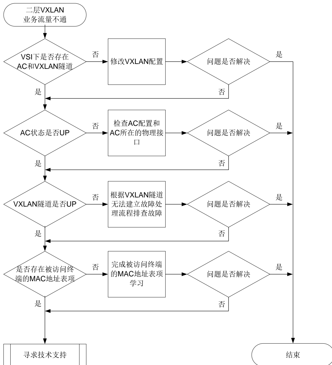
图13-3 二层 VXLAN 业务流量不通的故障诊断流程图
