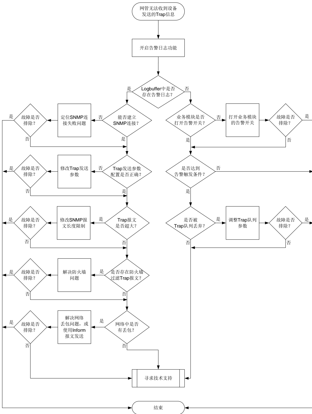
图18-6 网管无法收到设备发送的 Trap 的故障诊断流程图
