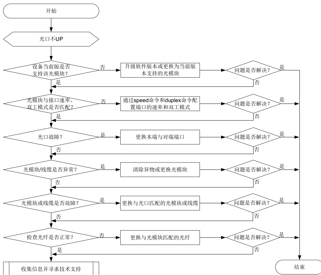
图2-21 故障诊断流程图
