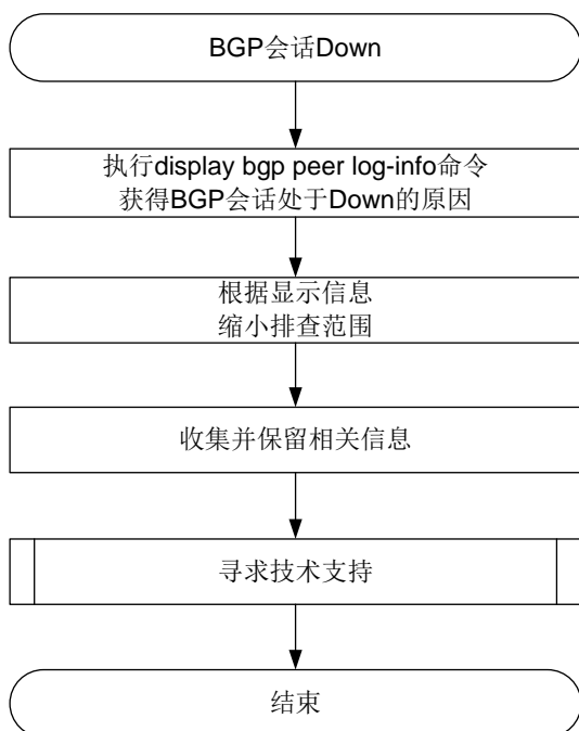
图8-2 BGP 会话 Down 的故障诊断流程图
