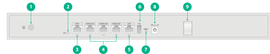
图1-3 ER3200G3 设备前面板
