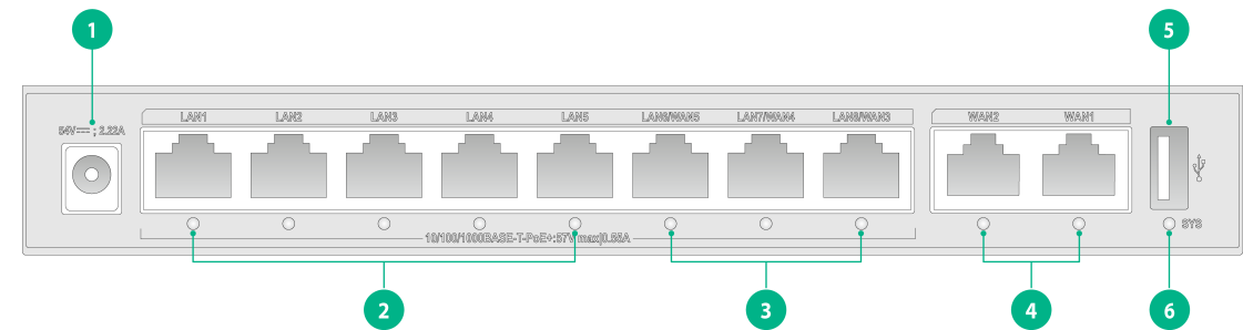
图1-9 ER3208G3-P-E 设备前面板
