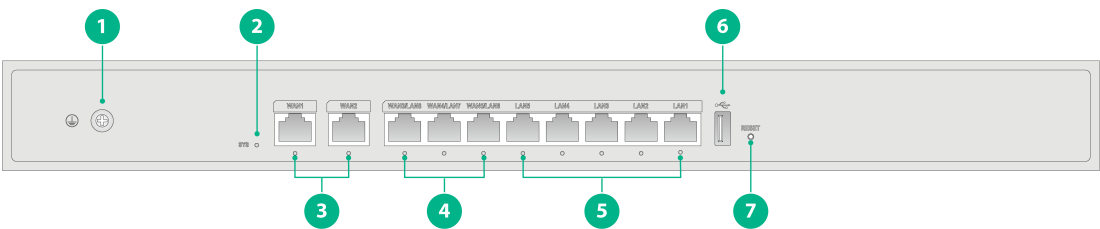
图1-12 ER3208G3-X 设备前面板
