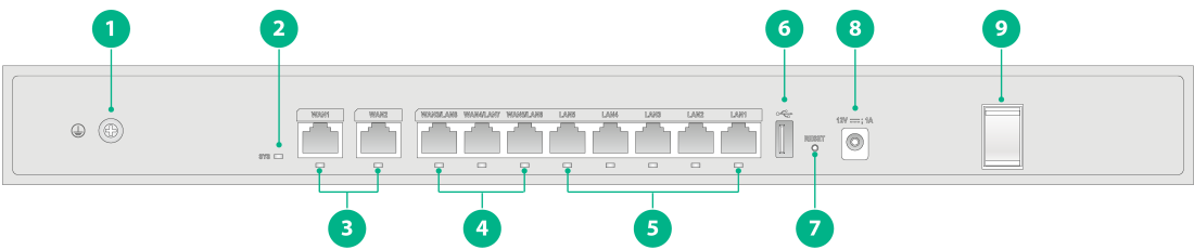
图1-6 ER3208G3 设备前面板
