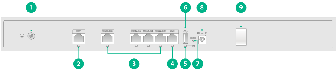
图1-14 ER3260G3 设备前面板
