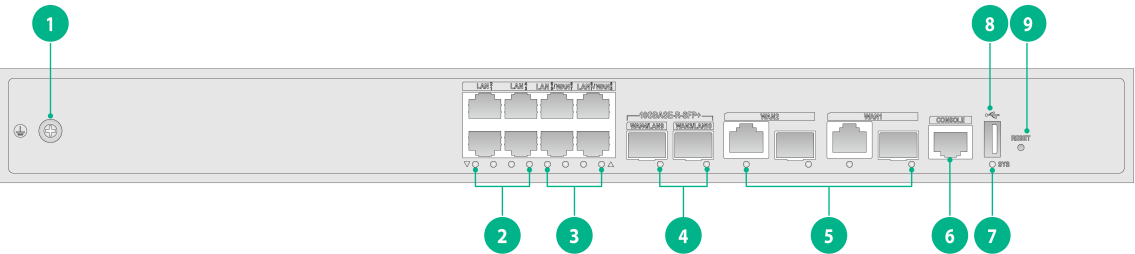
图1-20 ER6300G3 设备前面板
