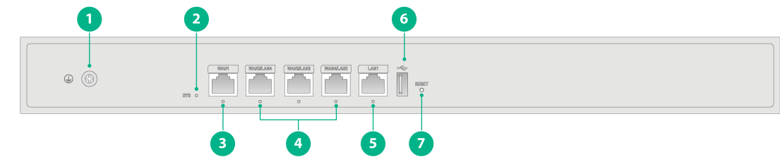
图1-4 ER3200G3-X 设备前面板
