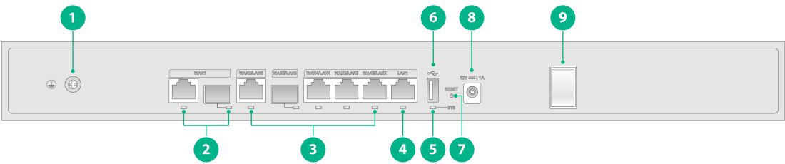
图1-17 ER5200G3 设备前面板
