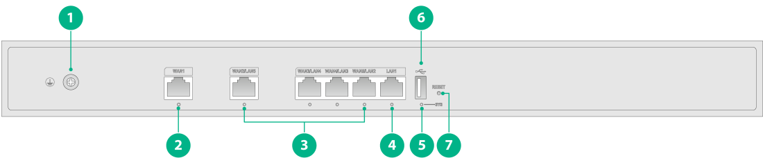
图1-15 ER3260G3-X 设备前面板
