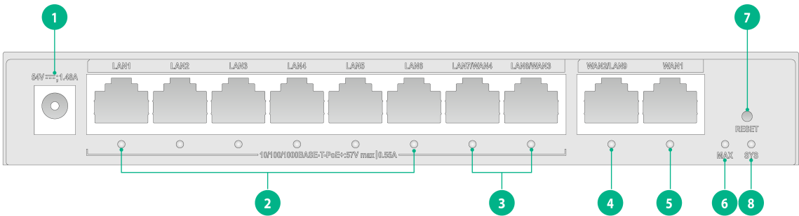
图1-7 ER3208G3-P 设备前面板
