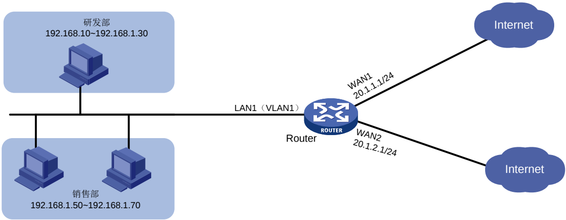
图1 策略路由典型配置组网图
