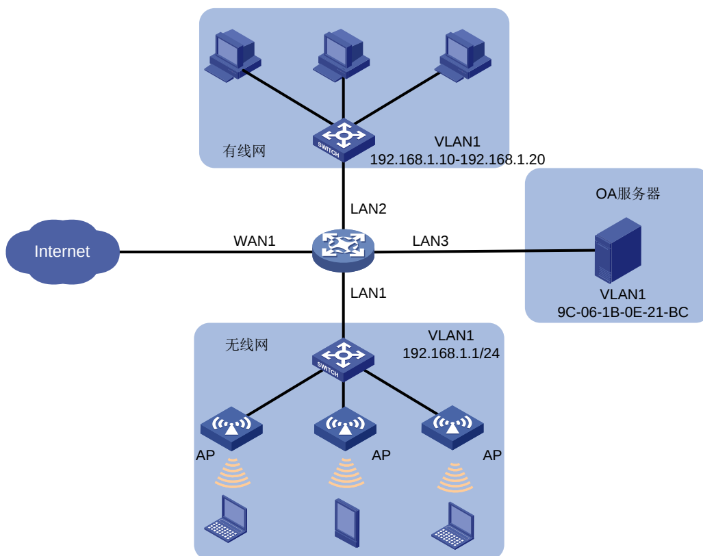
图1 Portal 认证典型配置组网图
