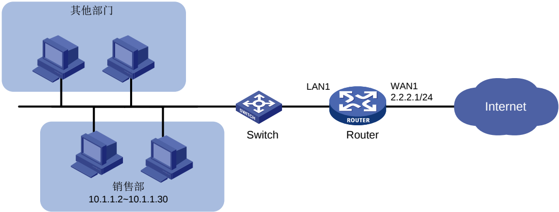
图14 网址黑名单典型配置组网图
