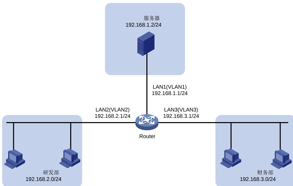
图1 防火墙典型配置组网图
