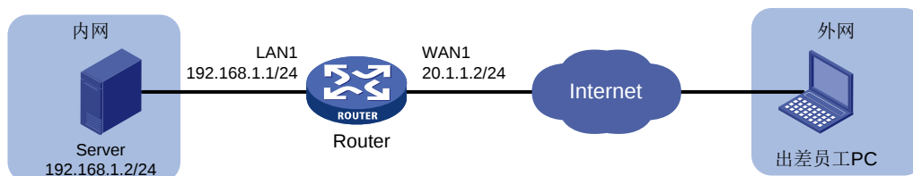
图1 端口映射典型配置组网图
