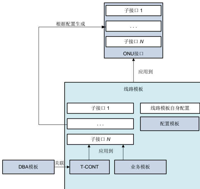
图35 ONU 配置下发时各类模板的关联关系
