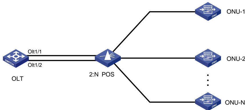
图36 单台 OLT 设备普通光纤备份组网示意图
