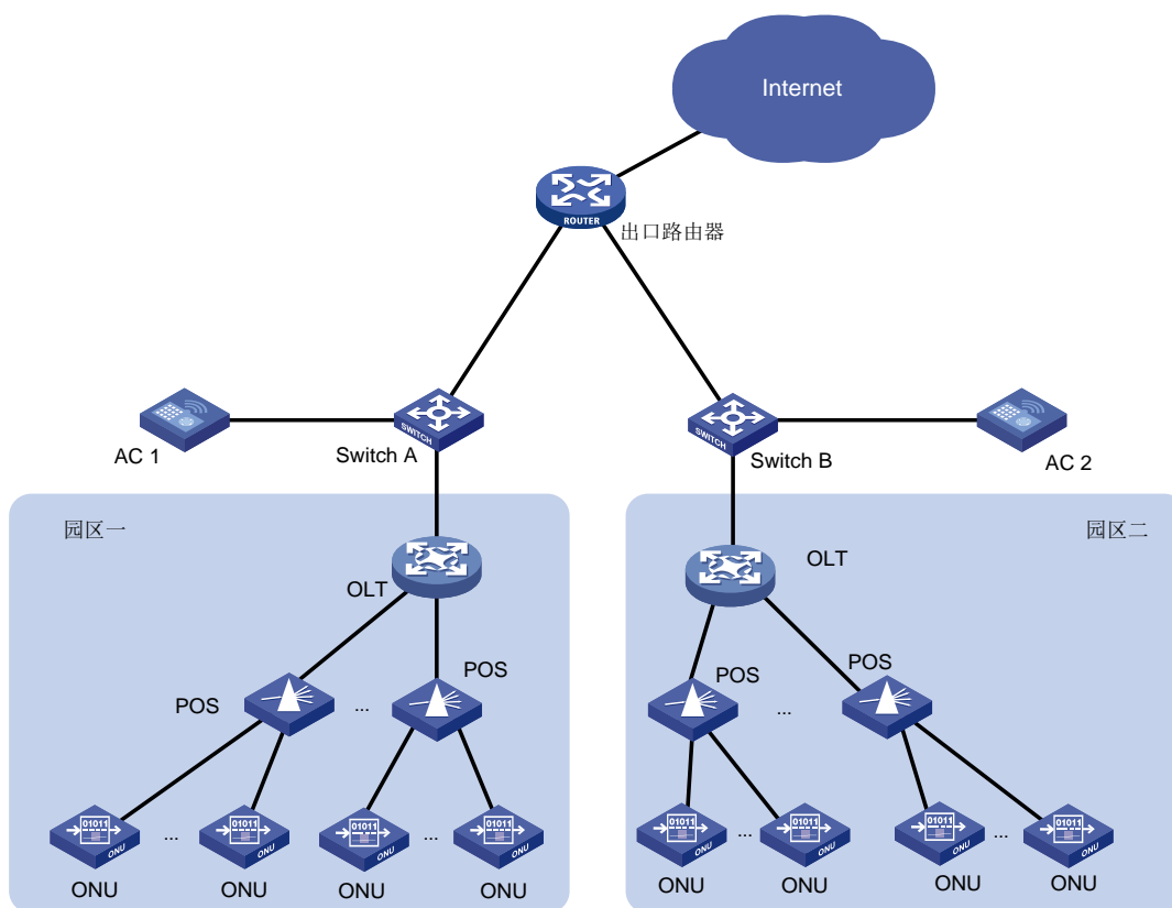
图34 园区网络组网图
