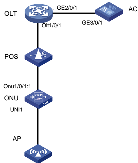
图4 EPON 教育网场景组网图
