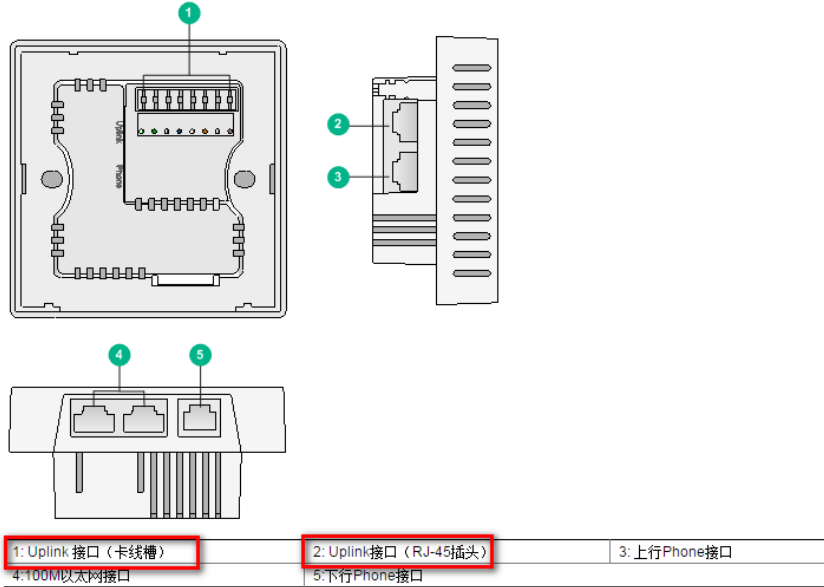
图A-2 WA2610H-GN(H2.0)无线接入点接口示意图
