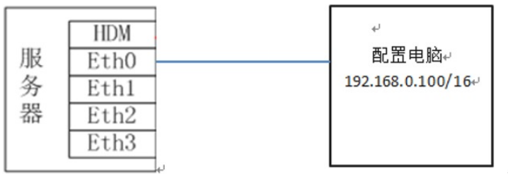
图2-2 配置电脑连接设备示意图
