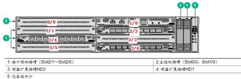
图A-2 F5030-D/F5060-D/F5080-D设备前视图
