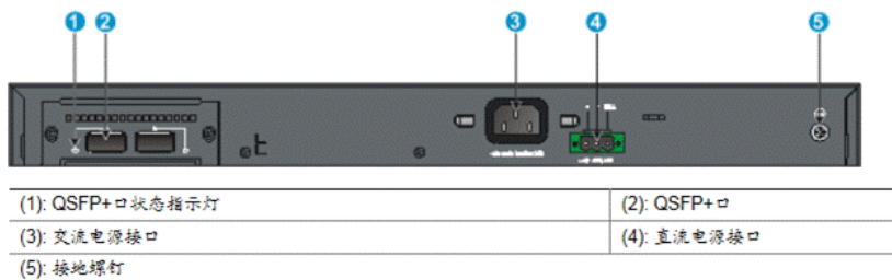
图1-4 S5560-54S-EI后面板示意图
