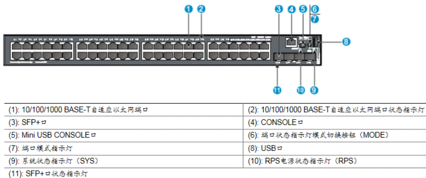
图1-4 S5560-54S-EI后面板示意图
