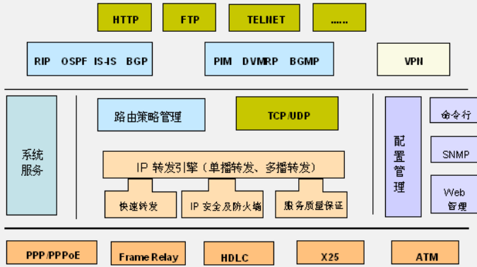
VRP体系结构图
