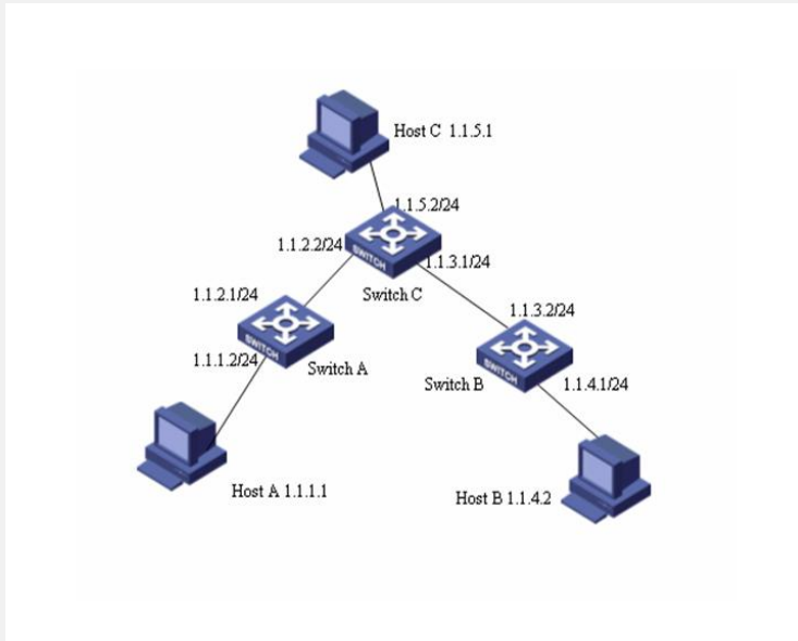
静态路由典型应用组网图
