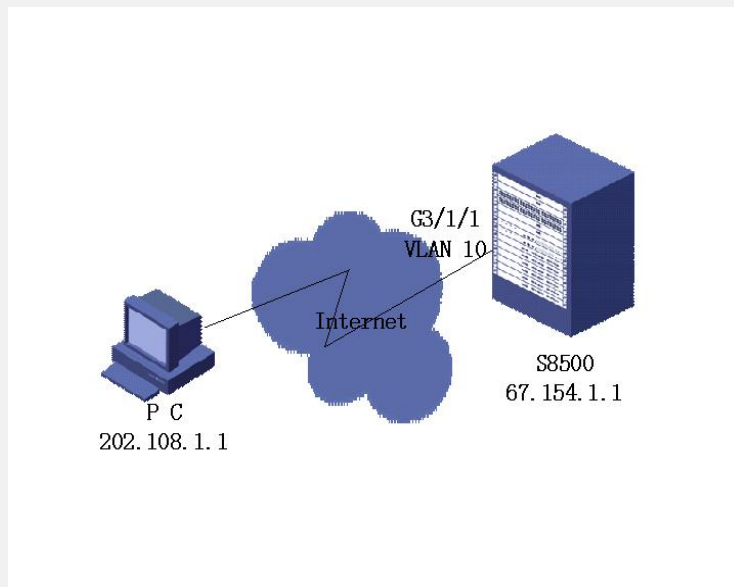
Telnet远程登录S9500典型应用组网图
