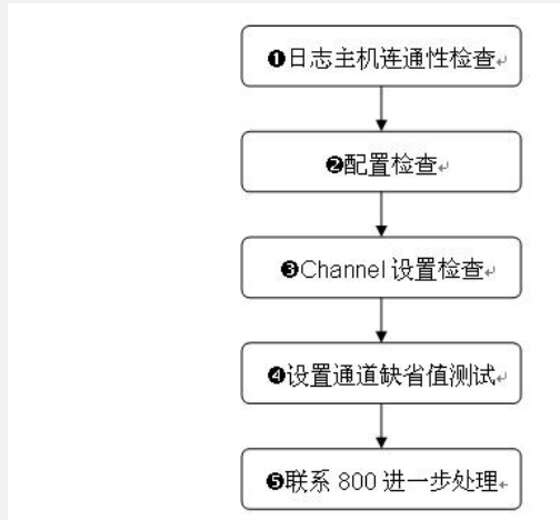
图一、日志主机 (loghost) 收不到信息故障处理流程
