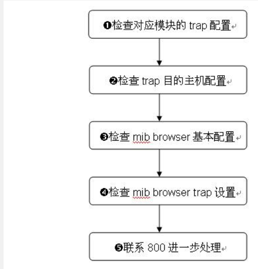
图一、mib-browser可以登陆S9500，但收不到TRAP故障处理流程
