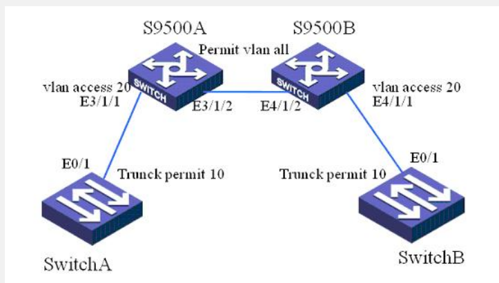
S9500交换机BPDU报文透传功能配置组网图
