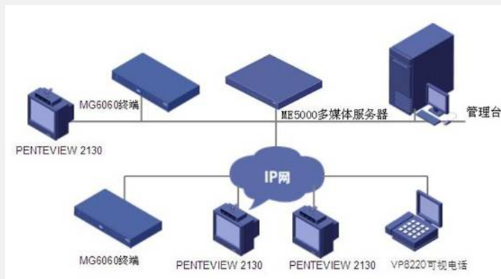
图1组网图
