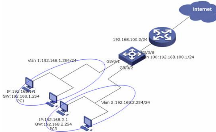
图一: vlan应用组网
