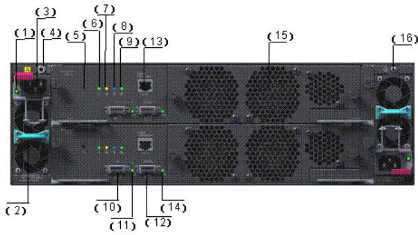
IX3040磁盘框前视图
