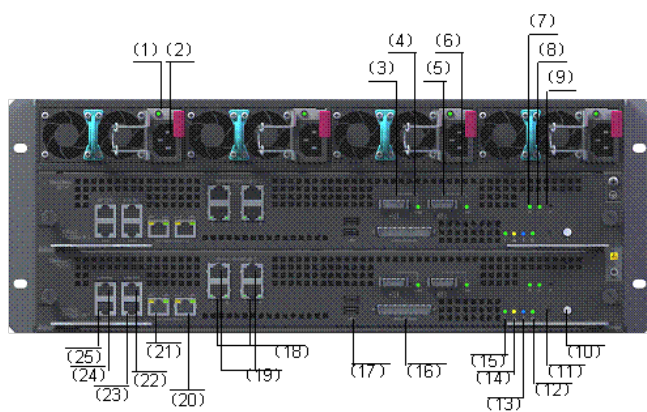
IX3040存储控制器前视图
