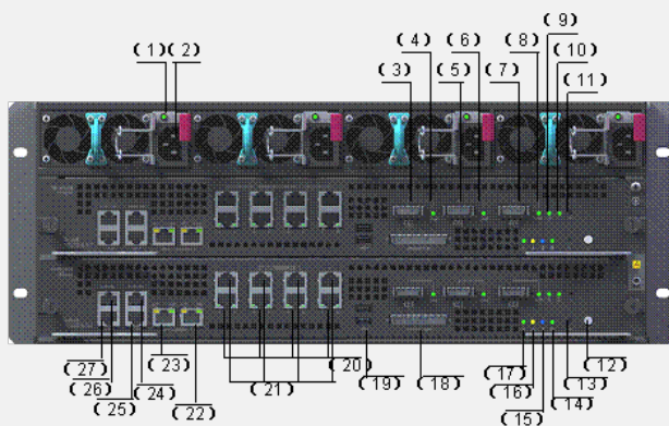
IX3080存储控制器前视图
